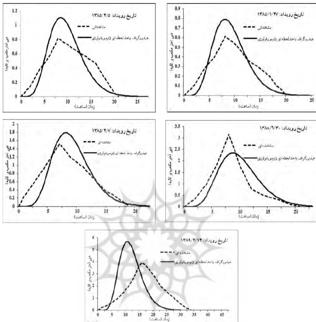
شکل (۲) مقایسه هیدروگراف‌های مدل هیدروگراف واحد لحظه‌ای ژئومورفولوژی و هیدروگراف‌های مشاهده‌ای متناظر
