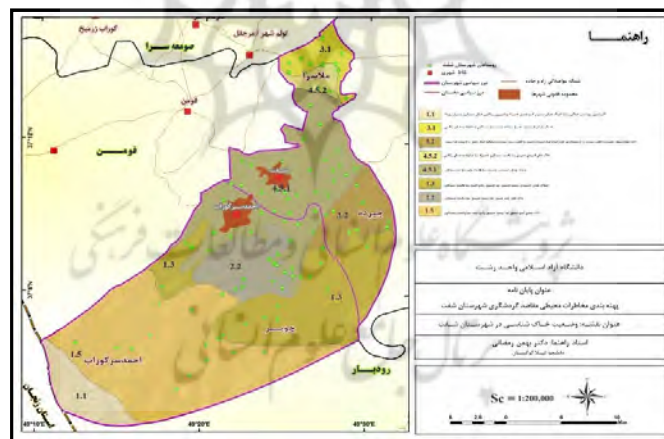
شکل ۴. نقشه وضعیت خاک شناسی شهرستان شفت (منبع: نگارندگان)
