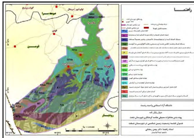
شکل ۳. نقشه وضعیت زمین شناسی (لیتولوژی) شهرستان شفت (منبع: نگارندگان)
