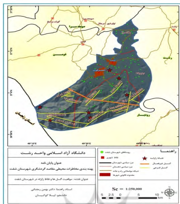
شکل ۶. نقشه وضعیت گسل ها و نقاط زلزله در شهرستان شفت (منبع: نگارندگان)
