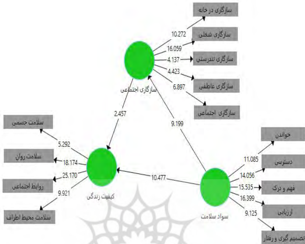
شکل ۲. نمودار معناداری ضرایب مدل معادلات ساختاری
