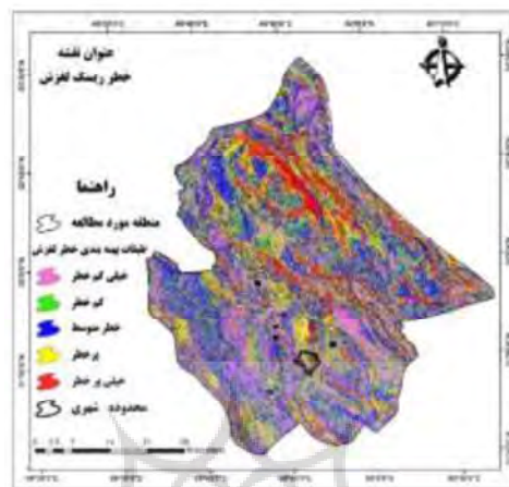
شکل ۴. نقشه پهنه‌بندی خطر زمین لغزش با عملکرد گامای فازی
