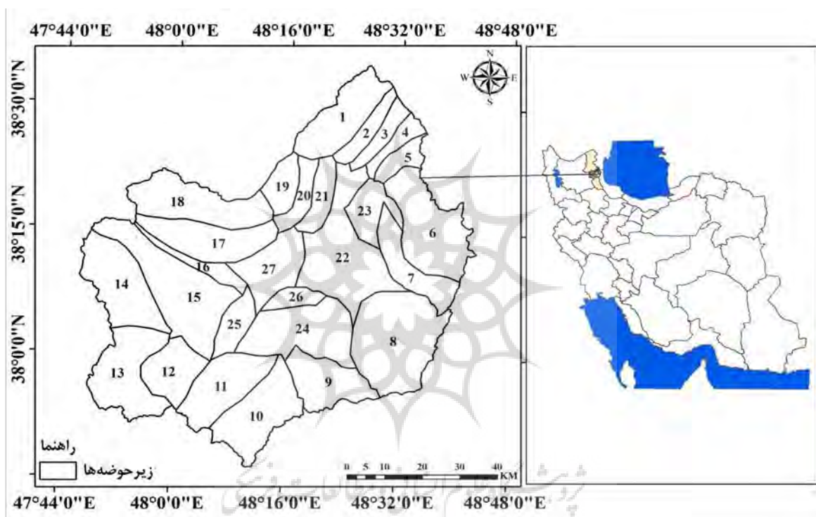
شکل (۱): موقعیت جغرافیایی زیرحوضه‌های آبخیز قره‌سو سامیان در استان اردبیل
