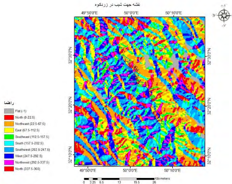
شکل ۶. نقشه جهت شیب در محدوده سیرک های یخچالی زردکوه
