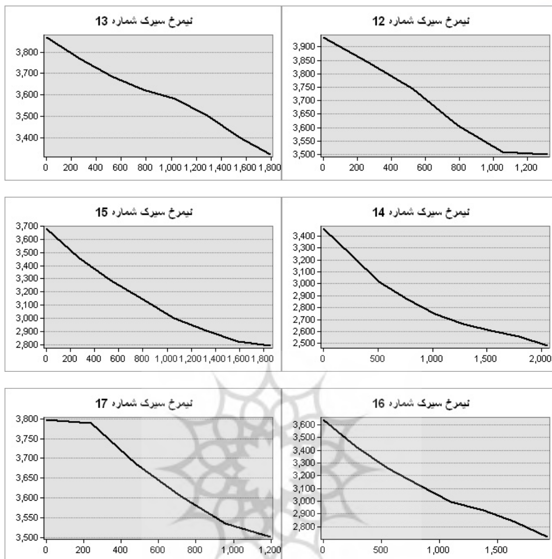
شکل ۷. نیمرخ طولی سیرک های یخچالی در محدوده ارتفاعات زردکوه
