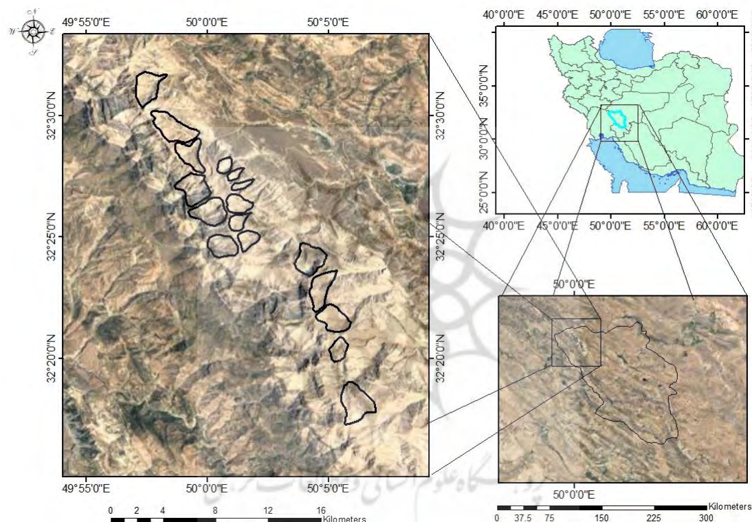
شکل ۱. موقعیت سیرک های یخچالی در ارتفاعات زردکوه بختیاری
