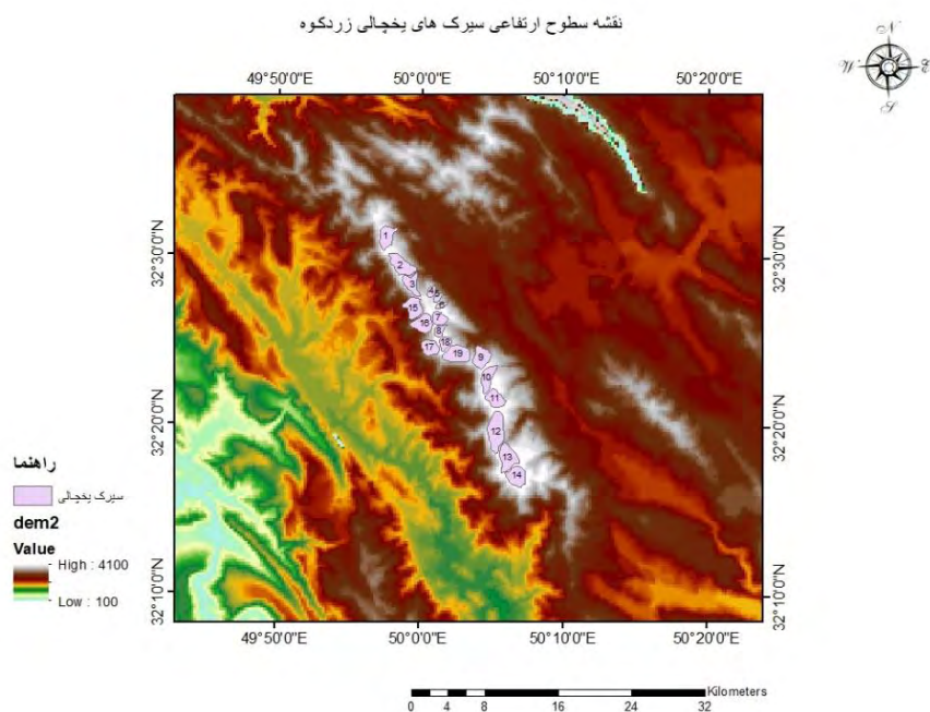
شکل ۴. نقشه سطوح رقومی ارتفاعی و موقعیت سیرک های یخچالی زردکوه
