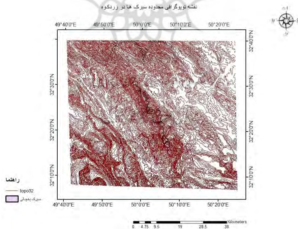
شکل ۳. نقشه توپوگرافی و موقعیت سیرک های یخچالی زردکوه
