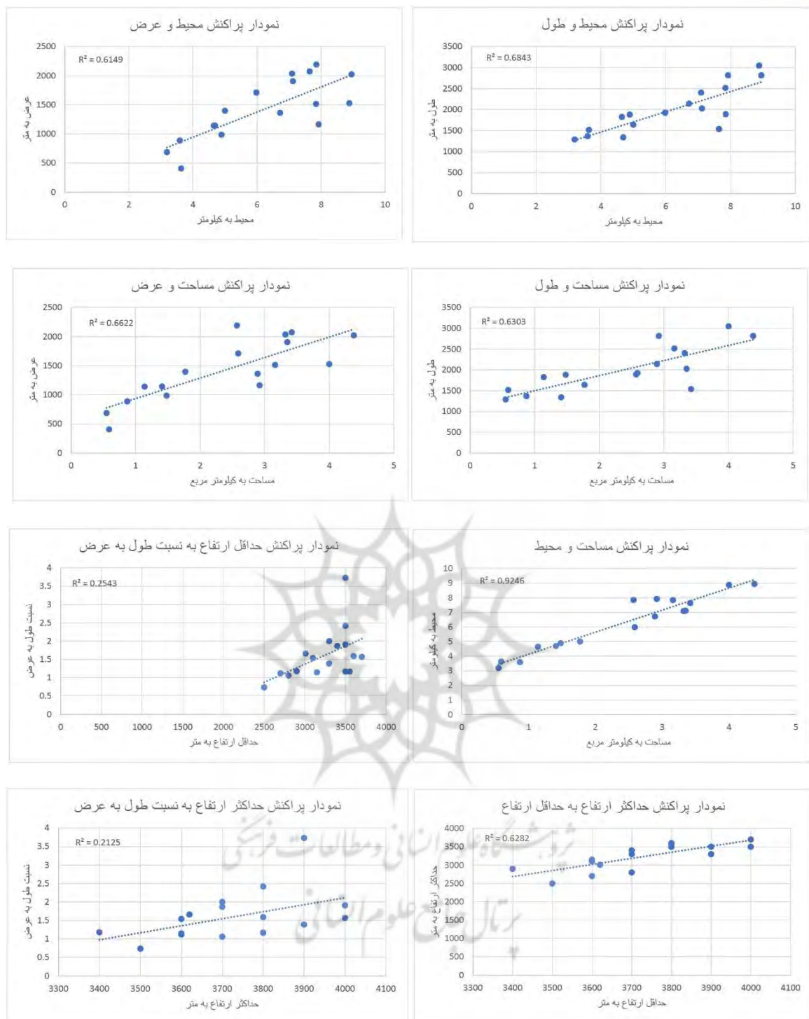
شکل ۸. نمودار پراکنش پارامترهای موثر در مورفومتری سیرک های یخچالی
