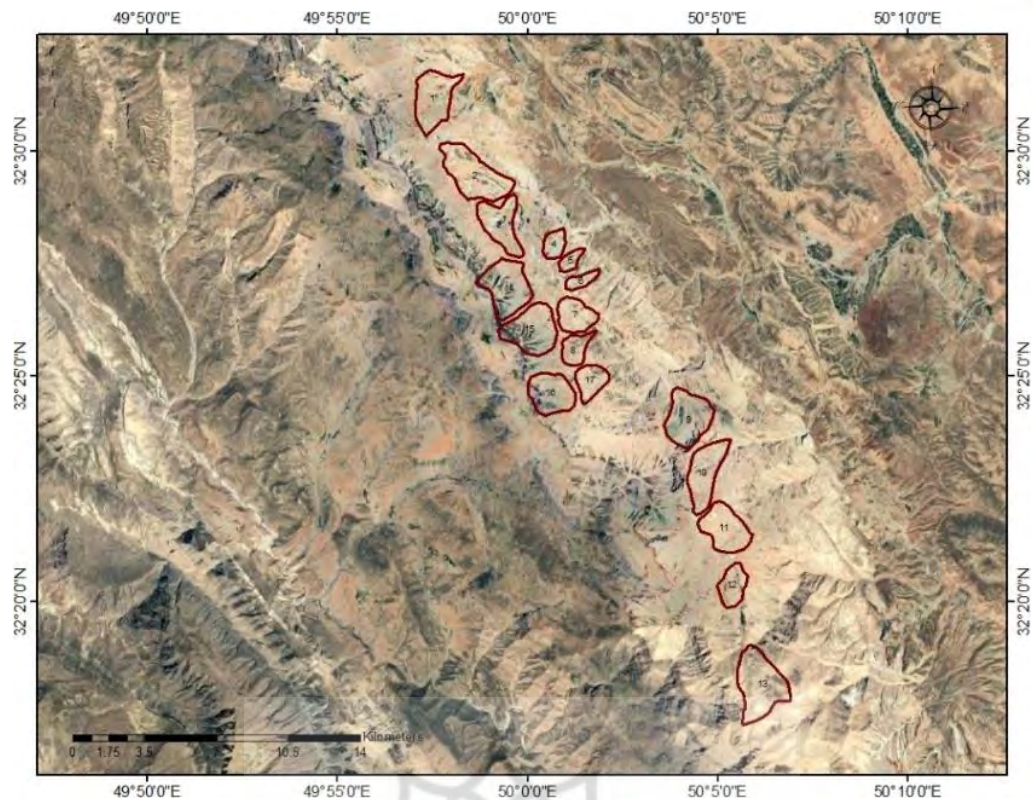
شکل ۲. موقعیت سیرک های یخچالی در زردکوه
