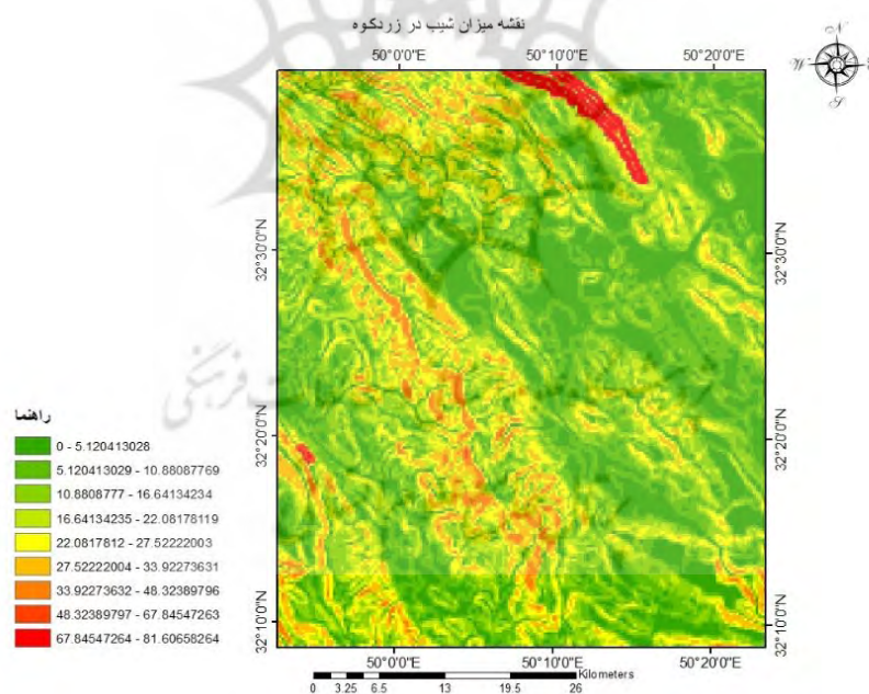
شکل ۵. نقشه میزان شیب در محدوده سیرک های یخچالی زردکوه
