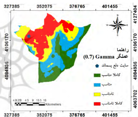
شکل ۲۵: عملگر گاما ۰/۷
