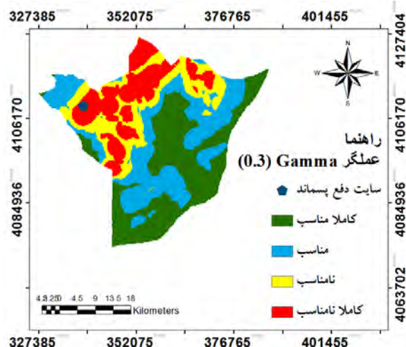
شکل ۲۳: عملگر گاما ۰/۳
