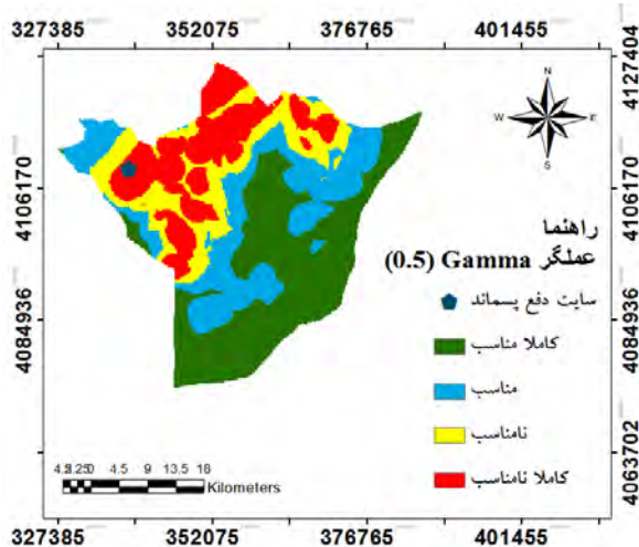
شکل ۲۴: عملگر گاما ۰/۵
