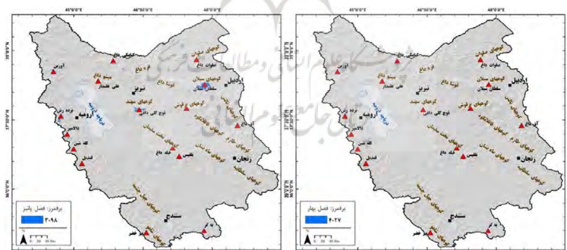
شکل (۲۱): پراکنش ارتفاع برف مرز در شمال غرب ایران (بهار) Figure (21): Snowline height distribution in northwest Iran (spring)
