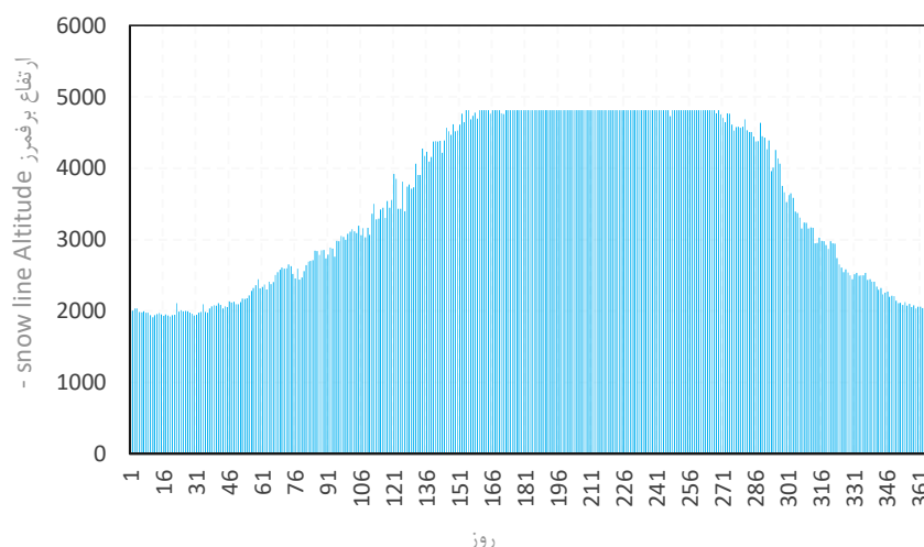
شکل (۲۶): میانگین ارتفاع برف مرز در شمال غرب ایران در بازه بلندمدت (۲۰۲۰-۲۰۰۳) (روش دوم) Figure (26): Average snow line height in northwest Iran in the long term (2003-2020) (Second Method)
