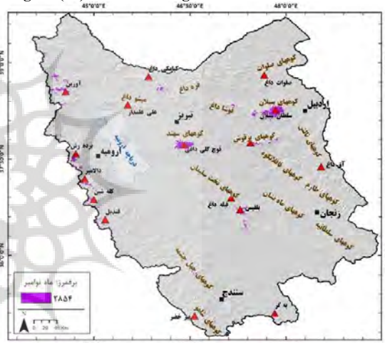
شکل (۱۶): پراکنش ارتفاع برف مرز در شمال غرب ایران (نوامبر) Figure (16): Snowline height distribution in northwest Iran (Nov)
