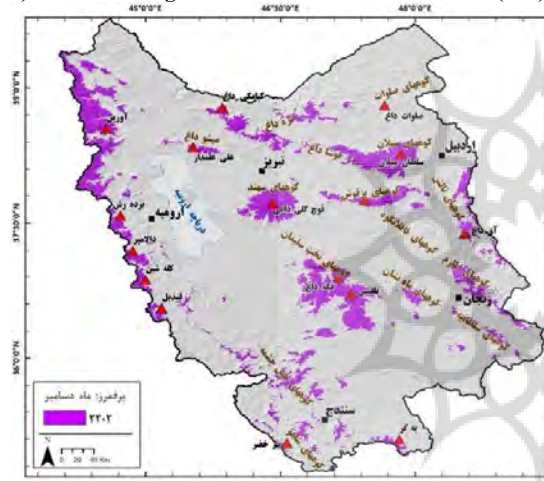
شکل (۱۷): پراکنش ارتفاع برف مرز در شمال غرب ایران (دسامبر) Figure (17): Snowline height distribution in northwest Iran (Dec)
