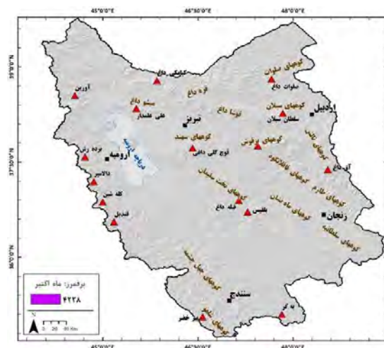
شکل (۱۵): پراکنش ارتفاع برف مرز در شمال غرب ایران (اکتبر) Figure (15): Snowline height distribution in northwest Iran (Oct)
