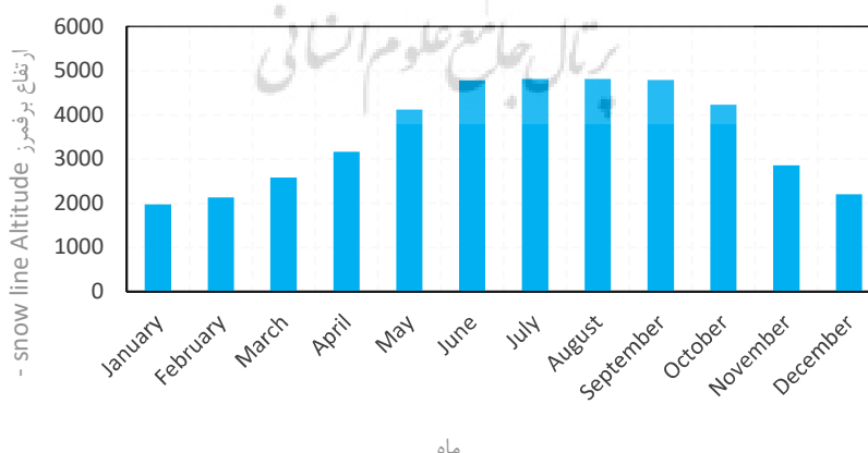
شکل (۱۸): میانگین ارتفاع برف مرز در شمال غرب ایران در ماه‌های مختلف سال (روش دوم) Figure (18): Average snowline height in northwest Iran in different months of the year (Second method)
