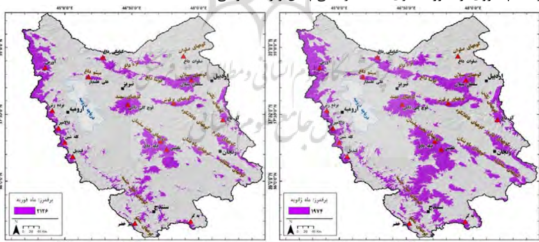
شکل (۷): پراکنش ارتفاع برف مرز در شمال غرب ایران (فوریه)
