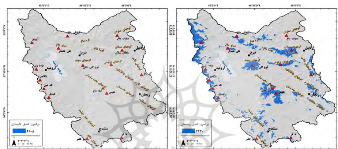
شکل (۱۹): پراکنش ارتفاع برف مرز در شمال غرب ایران (زمستان)
