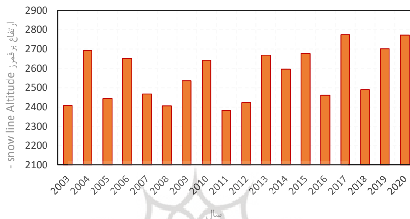
شکل (۴): میانگین ارتفاع برف‌مرز در شمال غرب ایران در بازه زمانی سالانه (روش اول)
