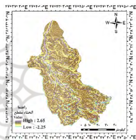
شکل ۱۱. نقشه شاخص انحناء مقطع (Profil Curvator) حوضه آبخیز مشکین چای
