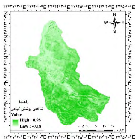
شکل ۲. شاخص پوشش گیاهی نرمال شده (NDVI) حوضه آبخیز مشکین چای
