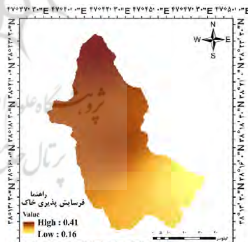
شکل ۱۳. نقشه عامل فرسایش‌پذیری خاک (K) حوزه آبخیز مشکین‌چای
