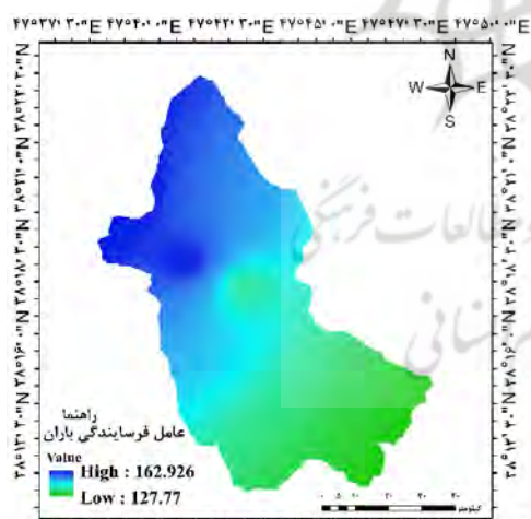
شکل ۱۲. نقشه عامل فرساینده باران (R) حوزه آبخیز مشکین‌چای
