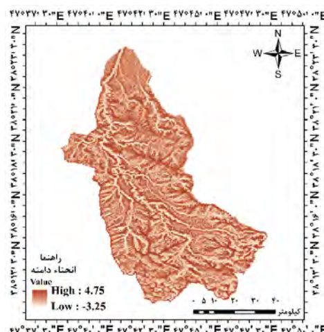
شکل ۹. نقشه شاخص انحناء دامنه (Curvator) حوضه آبخیز مشکین چای
