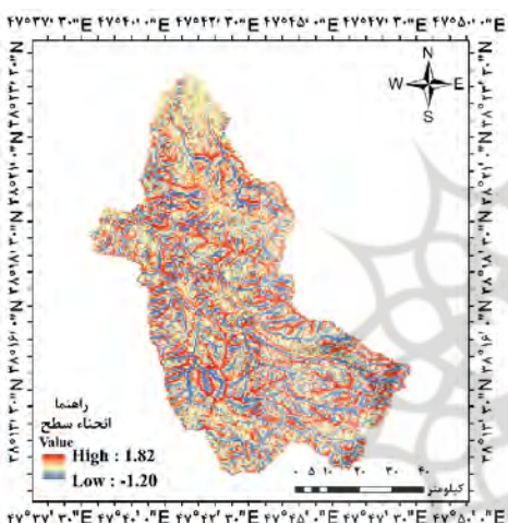
شکل ۱۰. نقشه شاخص انحناء سطح (Plan Curvator) حوضه آبخیز مشکین چای
