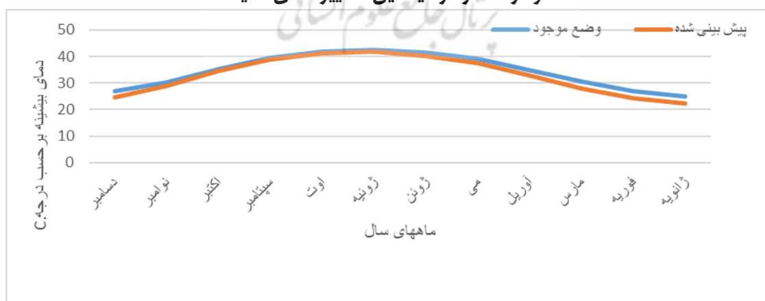
نمودار ۳. میانگین متغیر دمای بیشینه
