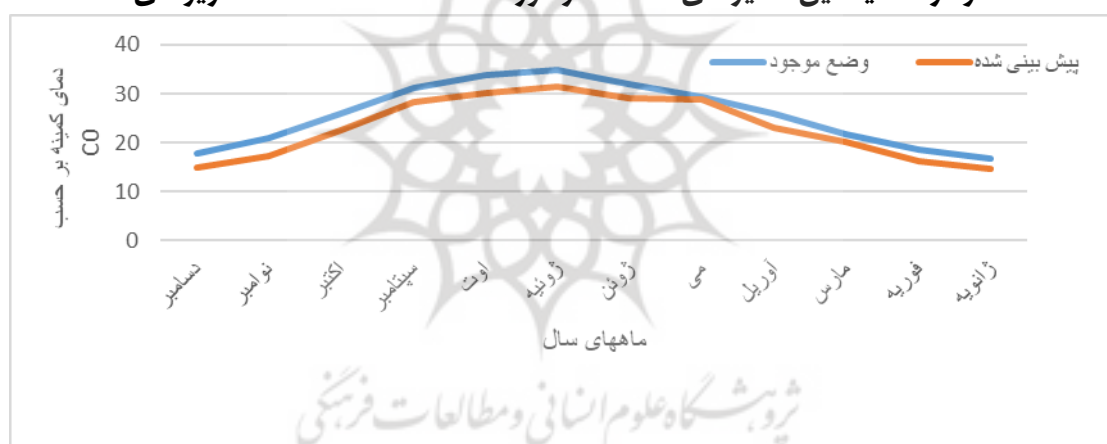
نمودار ۲. میانگین متغیر دمای کمینه
