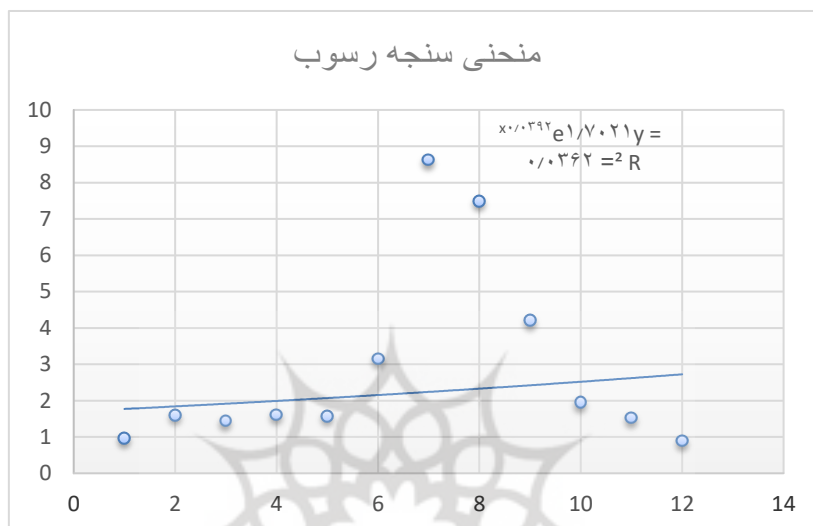
شکل ۴. منحنی سنج رسوب ایستگاه آبگرم حوزه گیوی چای
