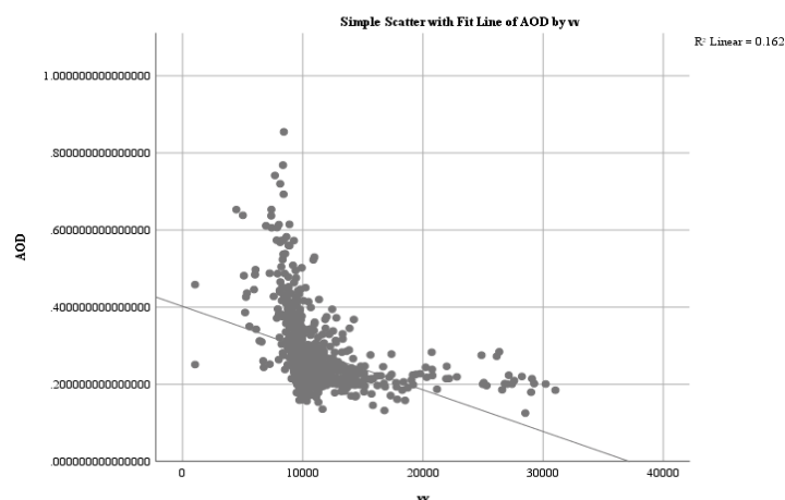
شکل ۲. نمودار پراکندگی بین AOD و دید افقی سال ۲۰۲۰ تا ۲۰۲۰
