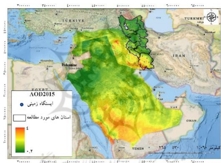
شکل ۱۰. میزان تغییرات گرد و غبار در سال ۲۰۱۵
