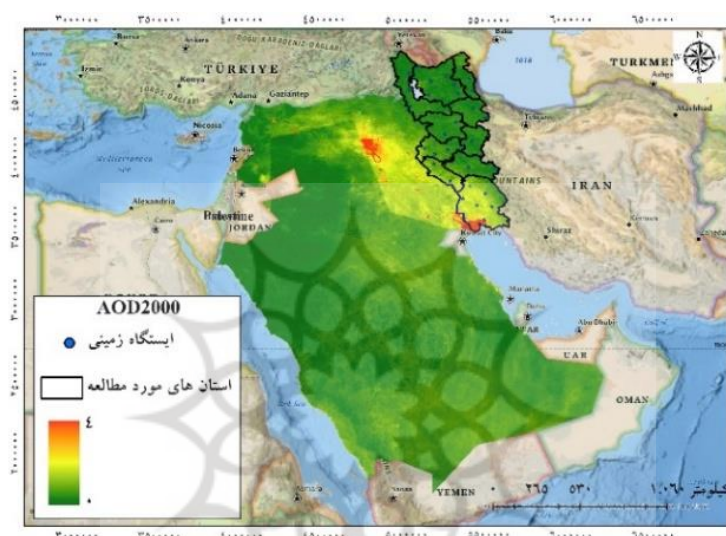
شکل ۷. میزان عمق اپتیک آئروسول در سال ۲۰۰۰
