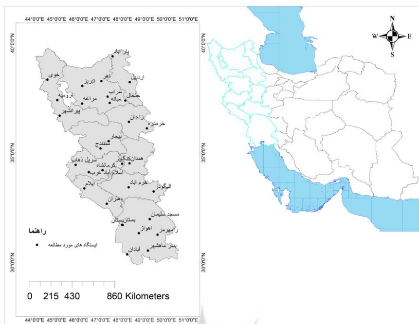
شکل ۱. نقشه پراکندگی ایستگاه‌های مورد مطالعه.
