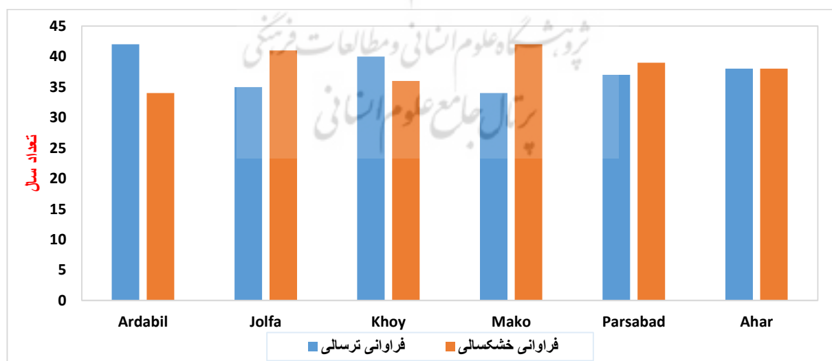
شکل ۵. نمودار مقایسه‌ای فراوانی ترسالی و خشک‌سالی در سال‌های دوره آینده در ایستگاه‌های حوزه ارس بر اساس شاخص SPI و خروجی مدل CNRM-CM6 تحت سناریوی SSP5-8.5
