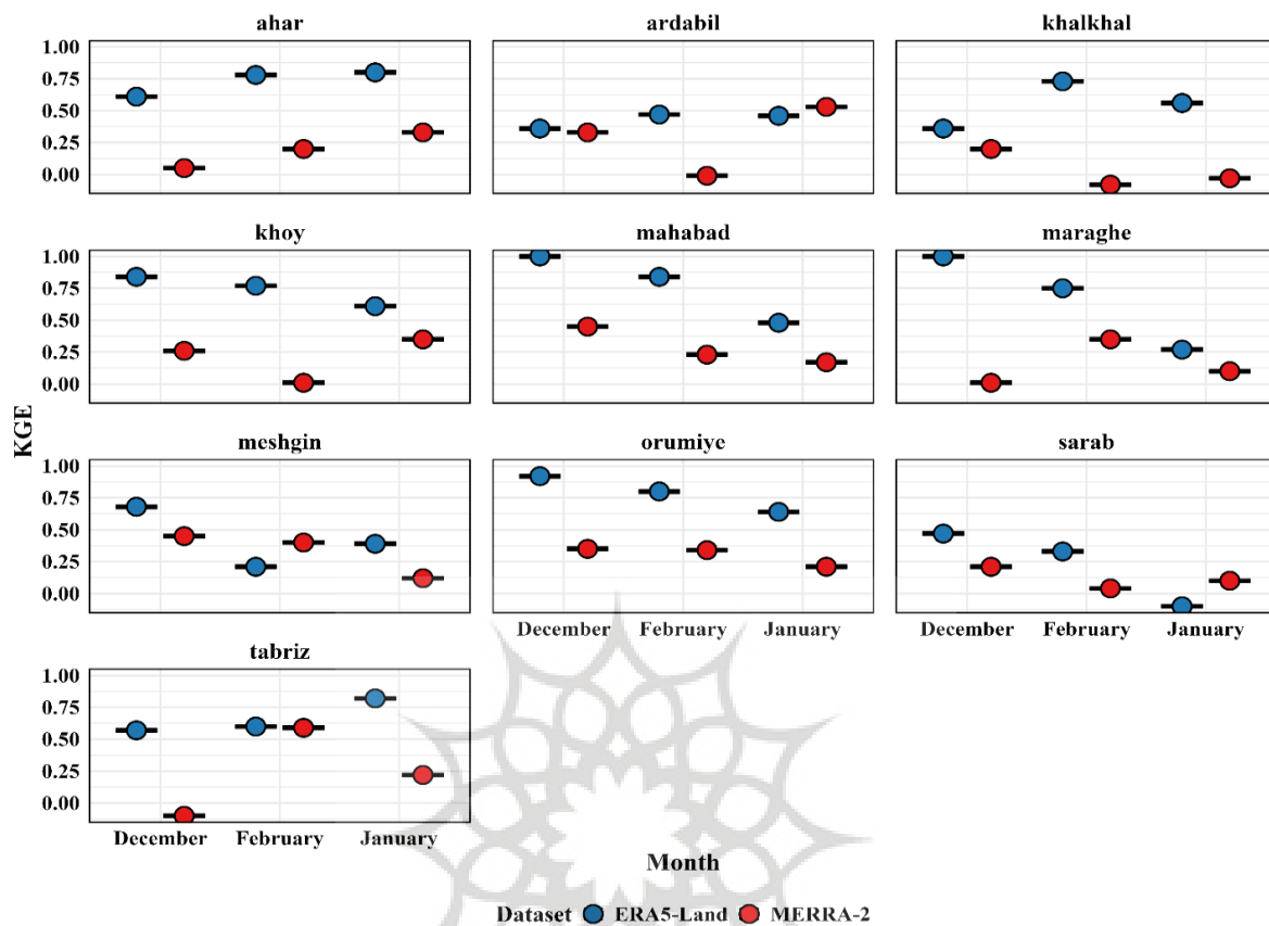
شکل ۶- نمودار جعبه‌ای عملکرد پایگاه‌های بازتحلیل در فصل زمستان، بر اساس شاخص KGE، برای ایستگاه‌های شمال غرب ایران در دوره ۲۰۰۴-۲۰۲۳
