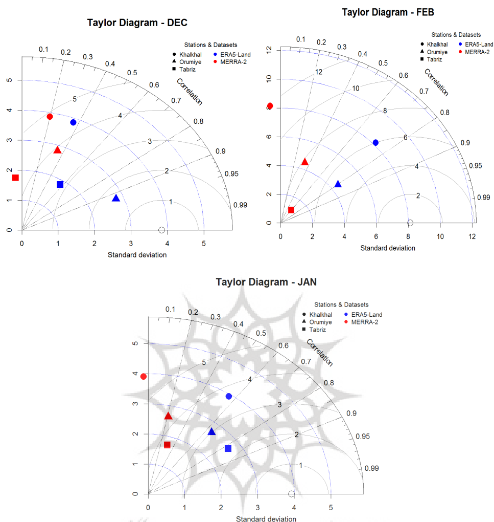
شکل ۳- نمودار تیلور ایستگاه‌های نماینده شمال غرب ایران جهت صحت سنجی برون‌داد مقیاس‌گاهی شده عمق برف توسط دو پایگاه بازتحلیل Fig. 3. Taylor diagram of representative stations in northwestern Iran for validating downscaled snow depth outputs from two reanalysis datasets
