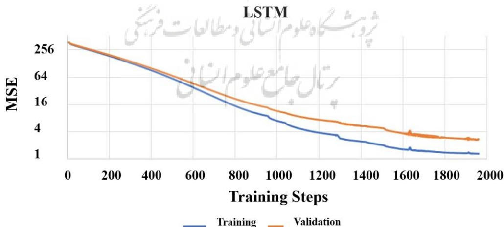
شکل ۱۰- منحنی یادگیری مدل LSTM بر اساس میانگین مربعات (MSE)
