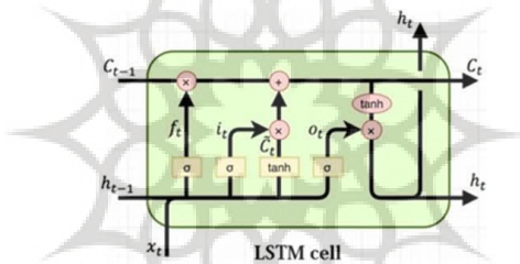
شکل ۷- ساختار داخلی سلول LSTM و نحوه جریان اطلاعات بین اجزای آن
