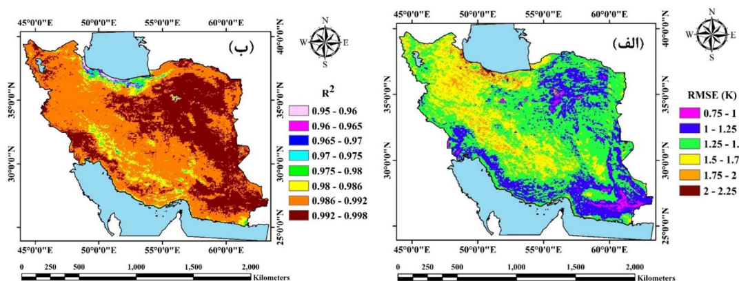
شکل ۷. نقشه خطای RMSE (الف) و ضریب تبیین (ب)، بین داده‌های موجود سری زمانی LST ساعتی سالیانه و داده‌های بازسازی شده با الگوریتم M-SSA
