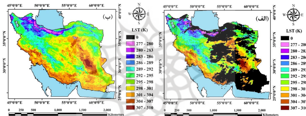
شکل ۸. نمونه‌ای از تصاویر با داده‌های از دست‌رفته (الف) و تصویر نظیر بازسازی از طریق الگوریتم M-SSA (ب)
