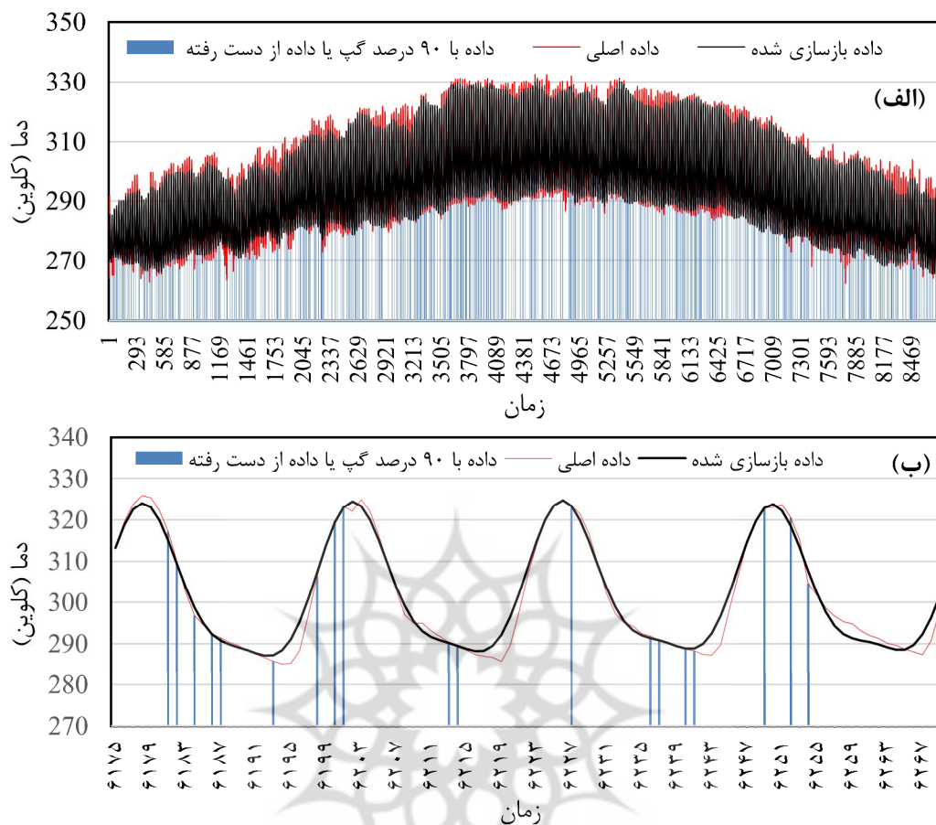
شکل ۱۲. یک نمونه سری زمانی LST ساعتی سالیانه (خطوط قرمز)، به همراه داده‌های از دست‌رفته مصنوعی با شدت ۹۰٪ (خطوط آبی) و سری زمانی بازسازی‌شده از طریق الگوریتم M-SSA (الف) و بزرگنمایی بخشی از سری زمانی (ب)
