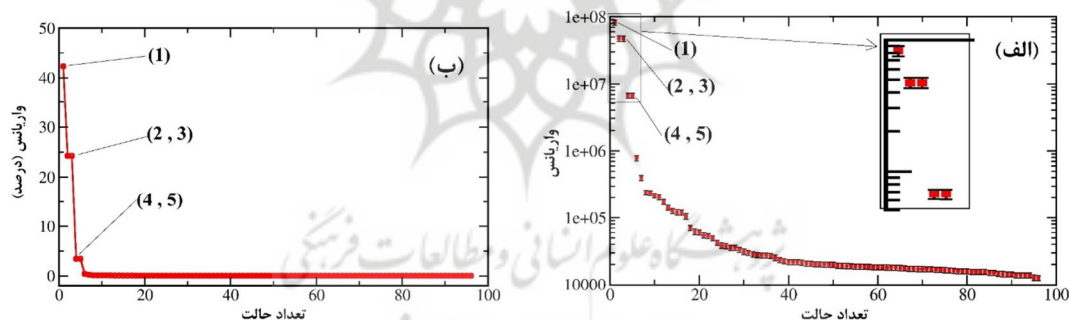
شکل ۴. منحنی اعداد تکین در پنجره ۹۶ ساعته (راست) و منحنی اعداد تکین نرمال شده (تغییرات واریانس نسبت به هر مؤلفه) در پنجره ۹۶ ساعته (چپ)
