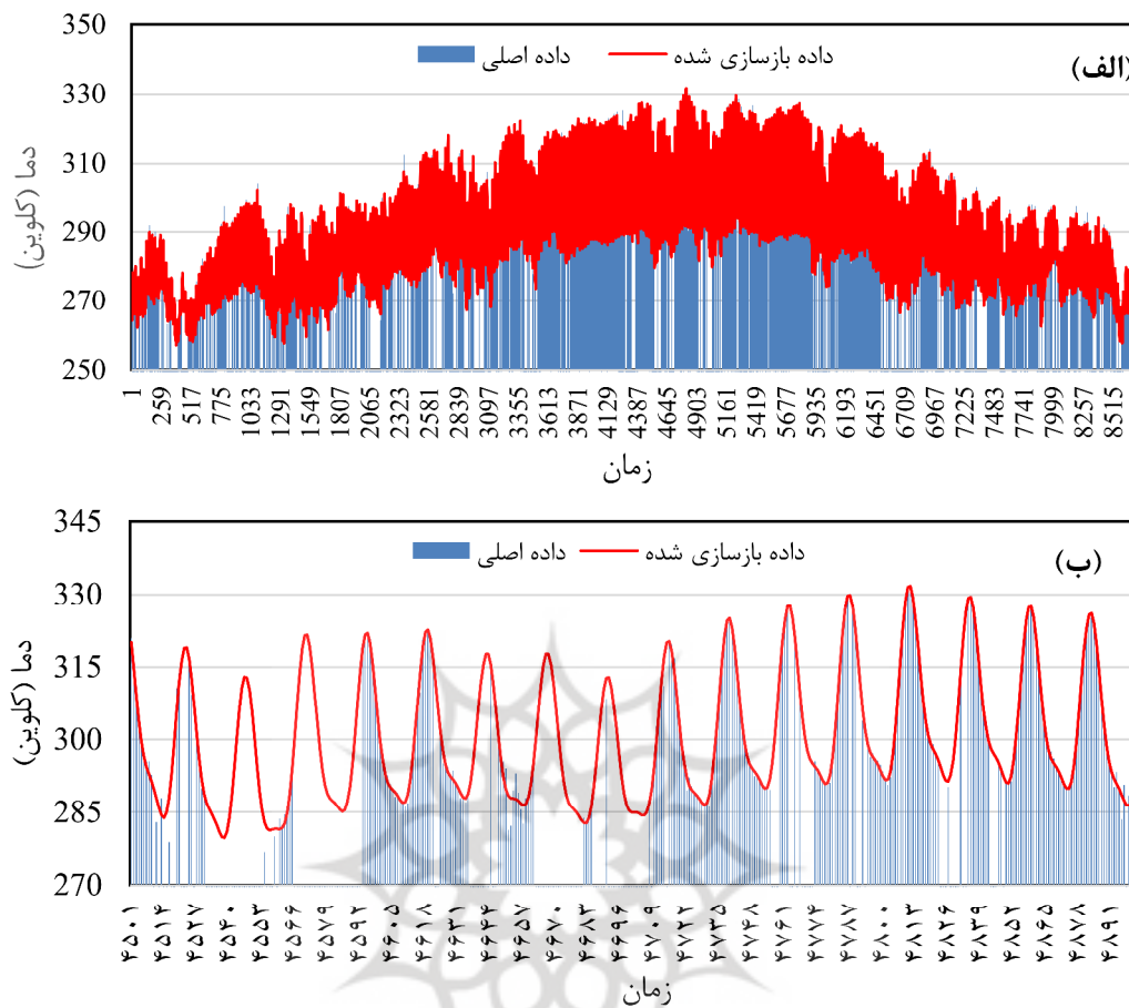
شکل ۹. نمونه سری زمانی LST ساعتی سالیانه (میللهای آبی)، با سری زمانی بازسازی شده (خط قرمز) از طریق الگوریتم M-SSA (الف) و بزرگنمایی بخشی از سری زمانی (ب)
