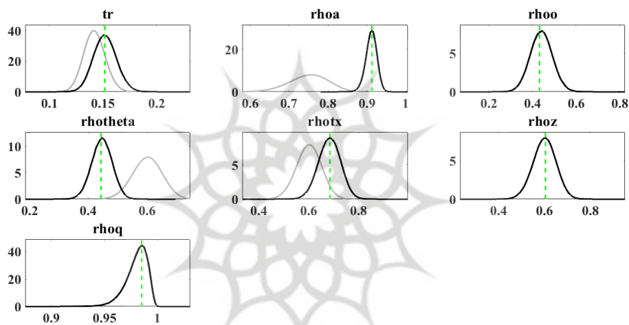
شکل ۲. توزیع‌های پیشین و پسین عواملی الگو
