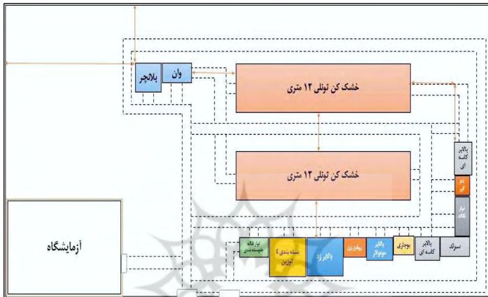
شکل (۳) نقشه چیدمان ماشین‌آلات خط تولید
