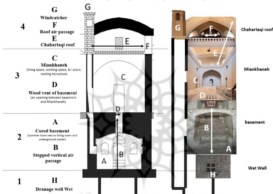
شکل ۴. شاکله مقطع اقلیمی در خانه‌ی توحیدی ۸
