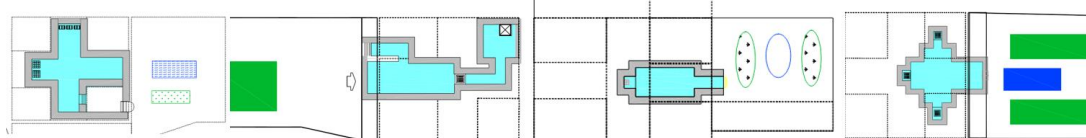
شکل ۳. اشکال مختلف زیرزمین در خانه‌های چهارصفه‌ی زواره و تناسب و موقعیت آنها نسبت به چهارصفه. (به ترتیب از راست به چپ: زیرزمین خانه طاهر خان نیری، طلایی، شفیی، هاشمی نسب)
