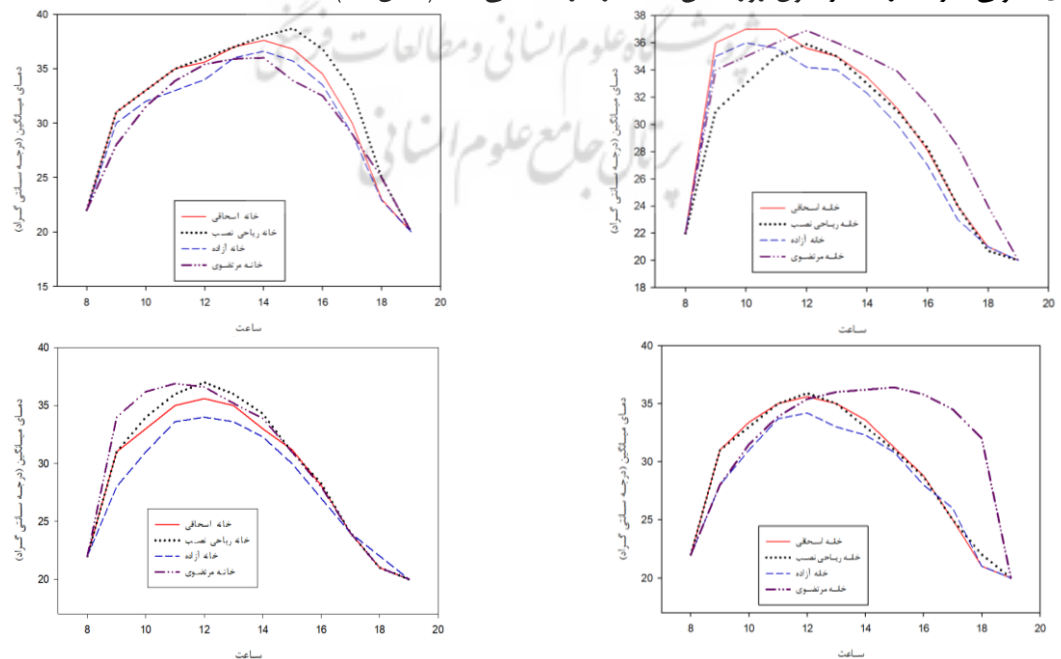
شکل ۱۳. نمودار دمای میانگین دیوار برای دیوارهای مختلف خانه‌ها در طول روز تابستان
