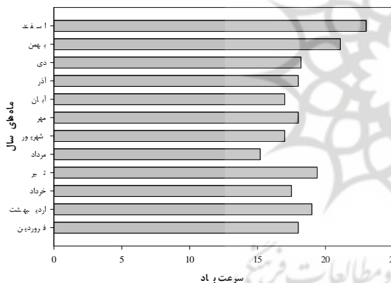
شکل ۳. نمودار داده‌های هواشناسی شهرستان شهرکرد در ده سال اخیر (سرعت باد در ماه‌های مختلف سال). منبع: اداره هواشناسی استان
