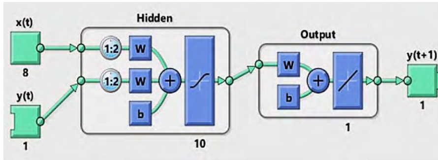
شکل (۲): معماری استاندارد شبکه نارکس
