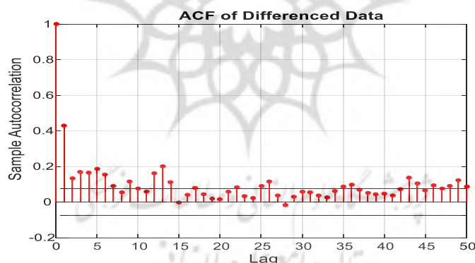
شکل (۵): نمودار خودهمبستگی داده‌های تفاضلی
