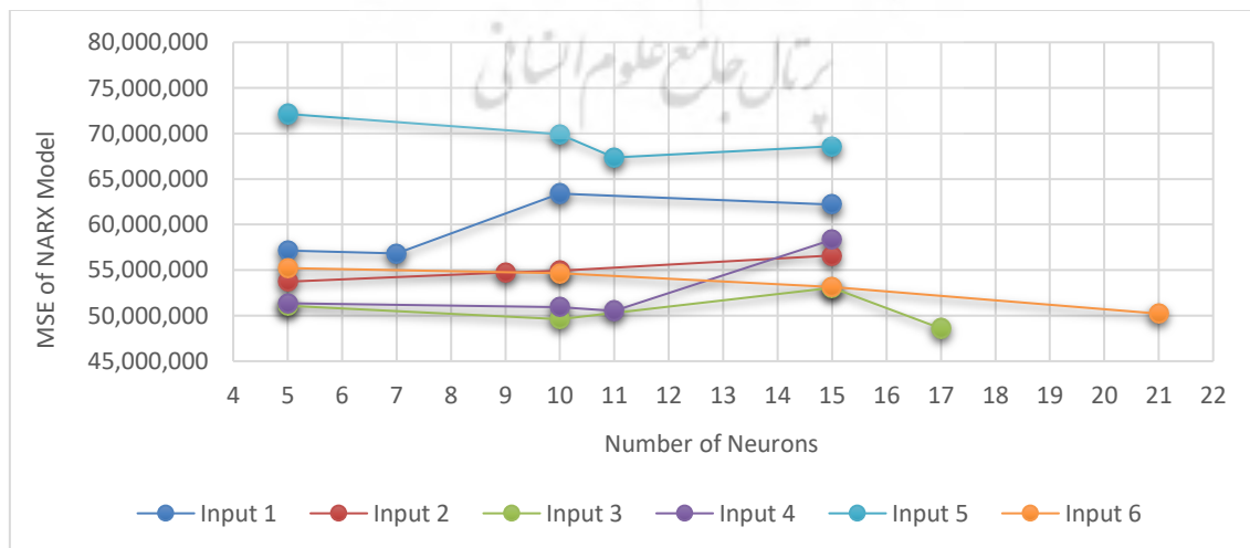
شکل (۴): تحلیل میزان حساسیت مدل نارکس به تعداد نورون ها
