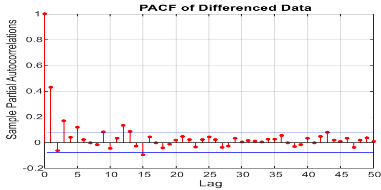
شکل (۶): نمودار خودهمبستگی جزئی داده‌های تفاضلی
