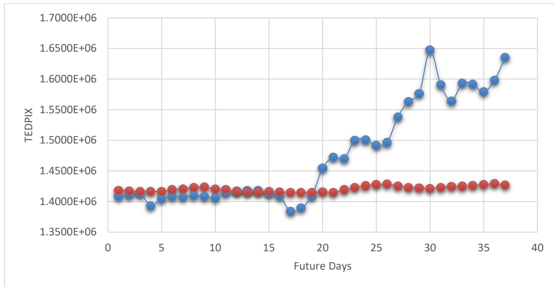
شکل (۳): مقایسه مقادیر پیش بینی شاخص در روزهای آتی (آبی رنگ) با داده های واقعی (نارنجی رنگ)
