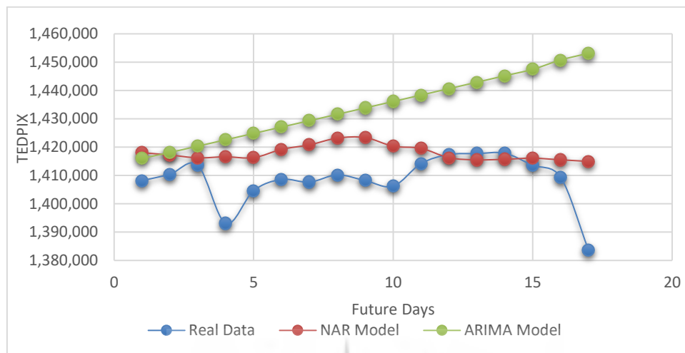
شکل (۷): مقایسه نتایج پیش‌بینی مدل آریمای با مدل نار و داده‌های واقعی
