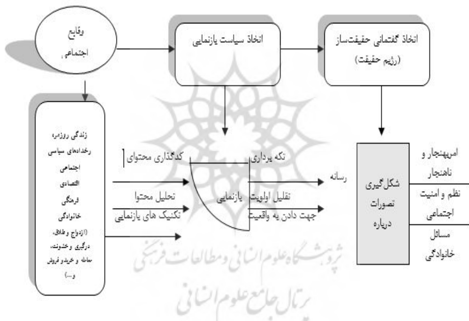
شکل ۱- مدل پژوهش
