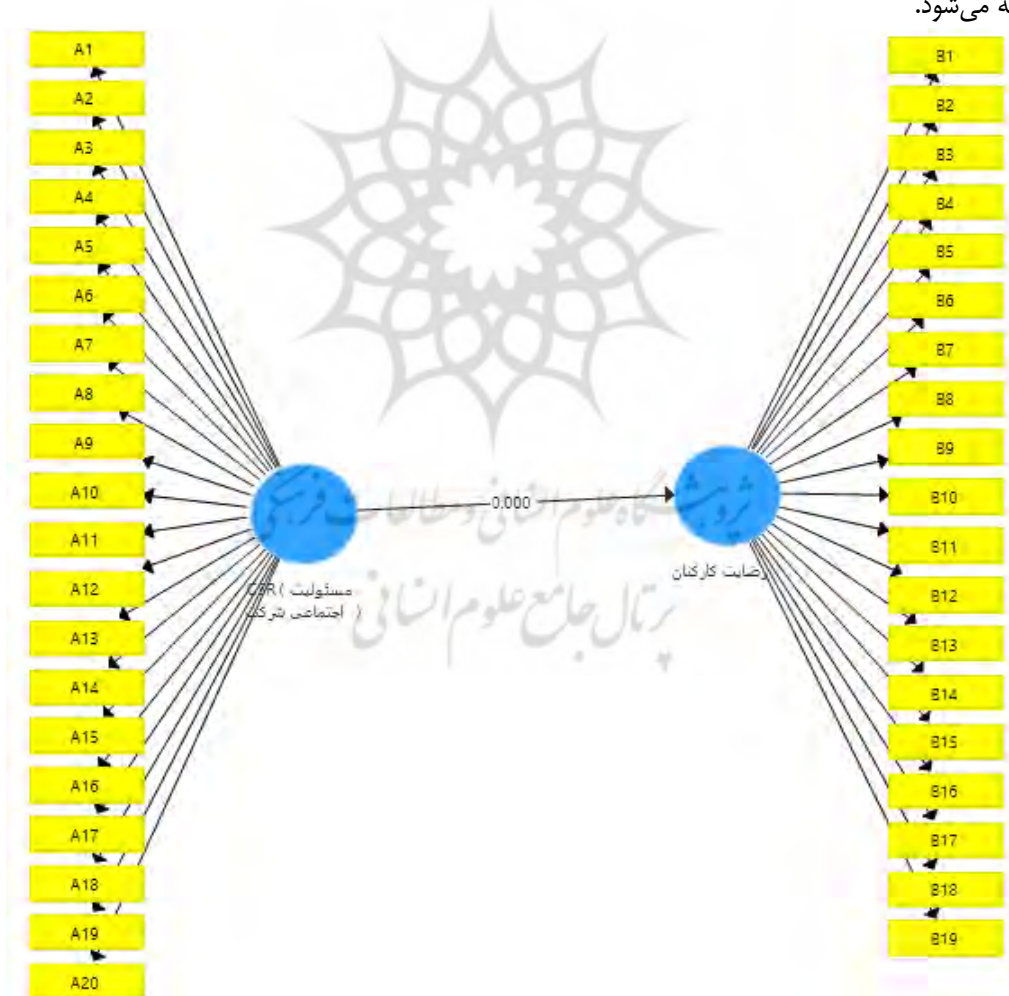
شکل ۲. معناداری (sig)
