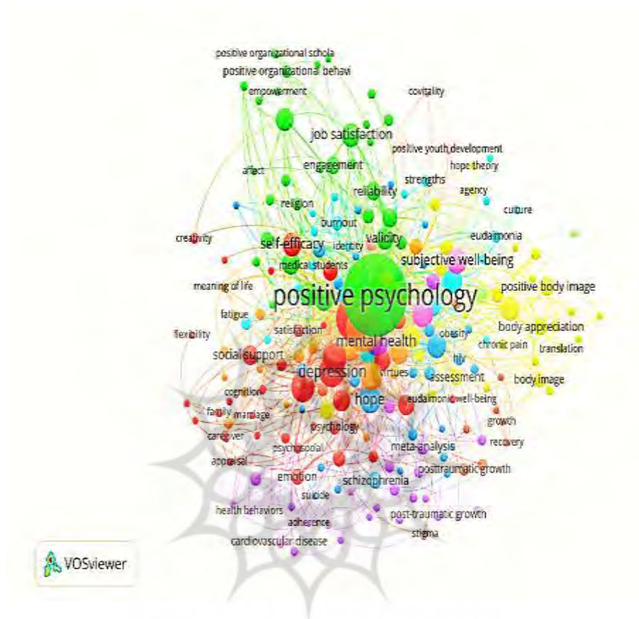
شکل ۱. شبکه هم‌رخدادی کلمات کلیدی توسط نویسندگان
