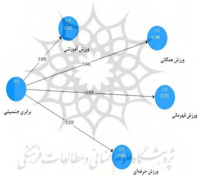
شکل ۲. مدل ساختاری پژوهش با ضرایب مسیر
