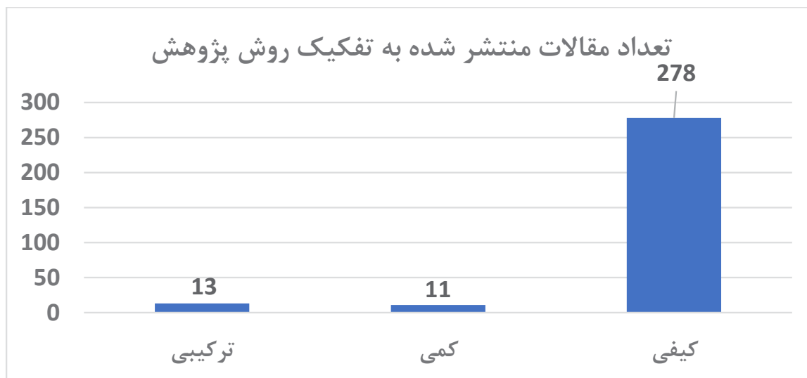
نمودار ۸: تعداد مقالات منتشر شده به تفکیک روش پژوهش (نگارندگان، ۱۴۰۳). Graph. 8: The Number of Articles Published by Research Method (Authors, 2024).
