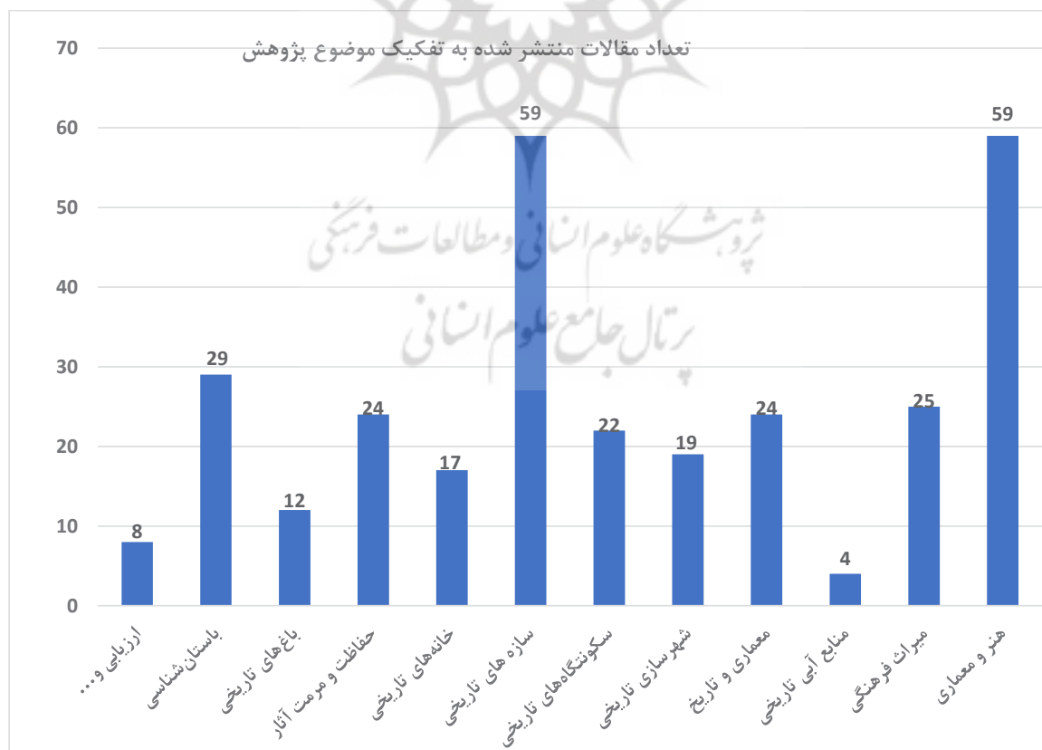
نمودار ۴: تعداد مقالات منتشر شده به تفکیک موضوع پژوهش (نگارندگان، ۱۴۰۳). Graph. 4: The Number of Articles Published by Research Topic (Authors, 2024).
