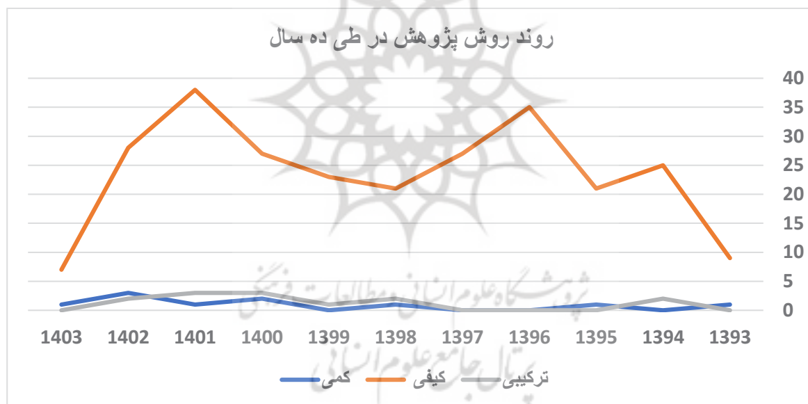
نمودار ۹: روند روش پژوهش در طی ۱۰ سال (نگارندگان، ۱۴۰۳). Graph. 9: Research Method Trends over a 10-Year Period (Authors, 2024).
