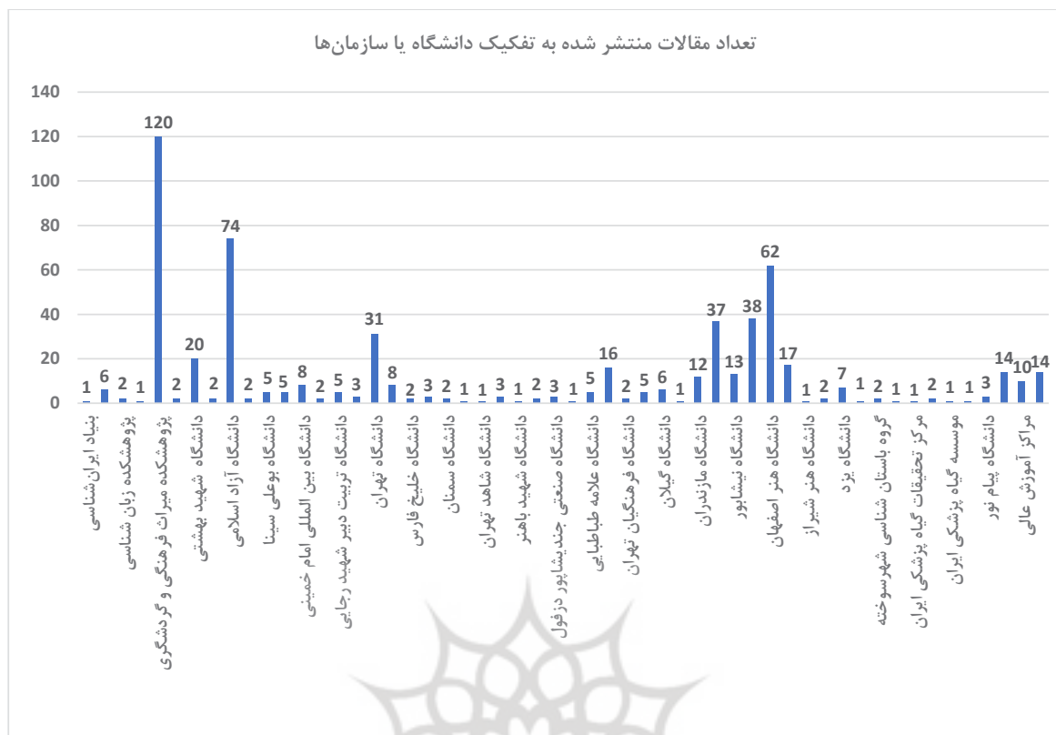
نمودار ۳: تعداد مقالات منتشر شده به تفکیک دانشگاه یا سازمان‌ها (نگارندگان، ۱۴۰۳). Graph. 3: The Number of Articles Published by Universities or Organizations (Authors, 2024).
