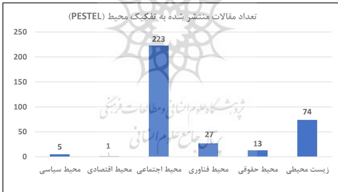
نمودار ۶: تعداد مقالات منتشر شده به تفکیک محیط (PESTEL)، (نگارندگان، ۱۴۰۳). Graph. 6: The Number of Articles Published by Environment (PESTEL), (Authors, 2024).
