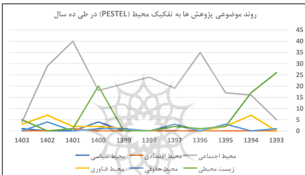
نمودار ۷: روند موضوعی پژوهش ها به تفکیک محیط (PESTEL) در طی ۱۰ سال (نگارندگان، ۱۴۰۳). Graph. 7: Thematic Trends of Research by Environment (PESTEL) over a 10-Year Period (Authors, 2024).
