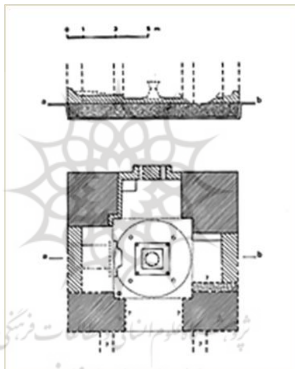
شکل ۱۴. پلان آتشکده مکشوفه از تورنگ تپه (Khosravi et al., 2018)
