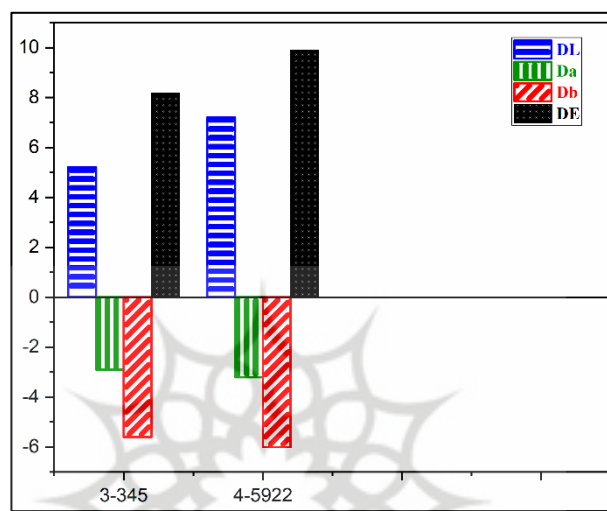
شکل ۴. نمودار تغییرات رنگی بین کاغذهای آهاردار و بدون آهار ۳۴۵-D و ۵۹۲۲-T
