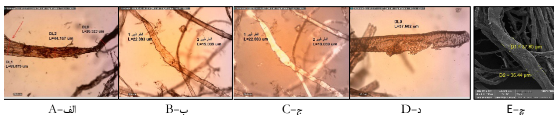
شکل ۵. الیاف پوستی و سلول‌های همراه شاهدانه در خمیر کاغذ ۳۴۵-D در بزرگنمایی ۱۰۰ X و ۲۰۰ X: (الف) و (ب) فیبرهای پوستی؛
