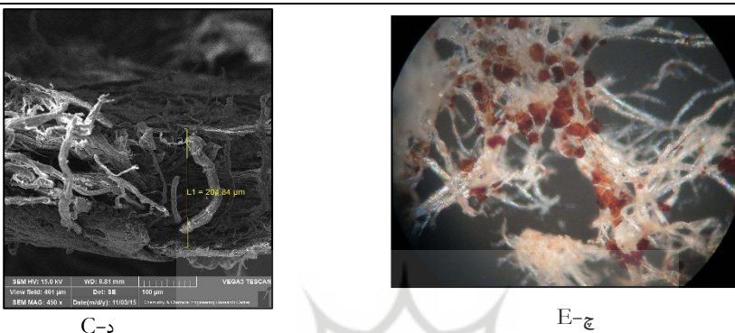
شکل ۲. کاغذ ترمه ۵۹۲۲- T: الف) کاغذ به رنگ قهوه‌ای؛ ب) عدم پراکندگی یکنواخت خمیر کاغذ، انحراف خطوط موازی قالب از راستای مستقیم، فاصله خطوط ۱-۱/۲ به تعداد ۷ عدد در ۱cm؛ ج) و د) لکه‌های قرمز رنگ، کاغذ به ضخامت ۰/۲۰ mm
