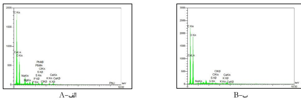
شکل ۱۱. نمودار آنالیز عنصری EDX: الف) کاغذ ۳۴۵-D؛ ب) کاغذ ۵۹۲۲-T
