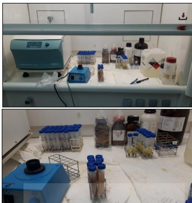
شکل (۳). آماده‌سازی نمونه‌های رسوب برای آنالیزهای ایزوتوپ اکسیژن ۱۸
