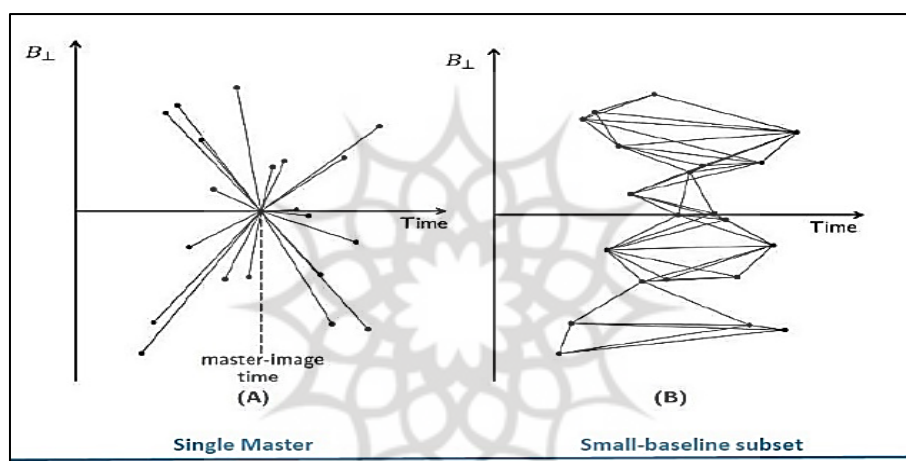
شکل (۲). (A) روش تک مرجعی و (B) خط مبنای کوتاه (آجورلو، ۱۳۹۷: ۳۳)
