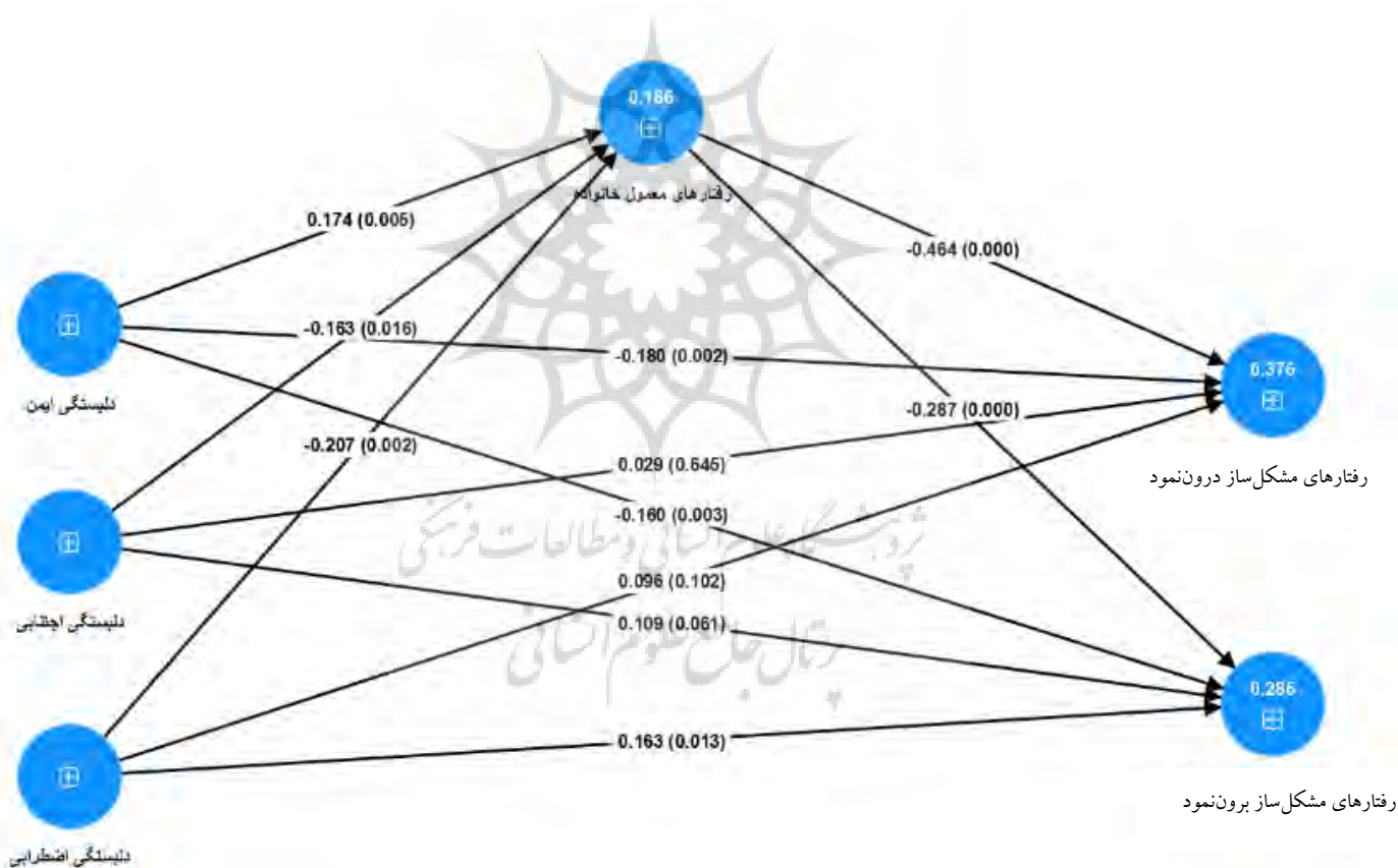
شکل ۲: ضرایب مسیر بین متغیرها و سطوح معناداری
