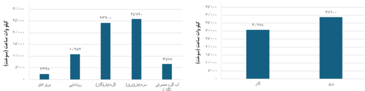
شکل ۶: الگوی مصرف انرژی سالانه ساختمان مرجع (بدون سیستم های سبز)
