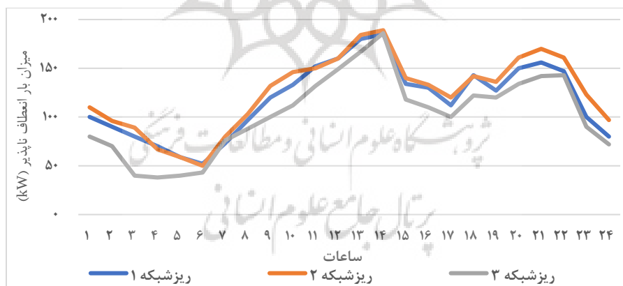
شکل ۷ میزان بار انعطاف‌ناپذیر در سیستم ریزشبکه چندگانه
