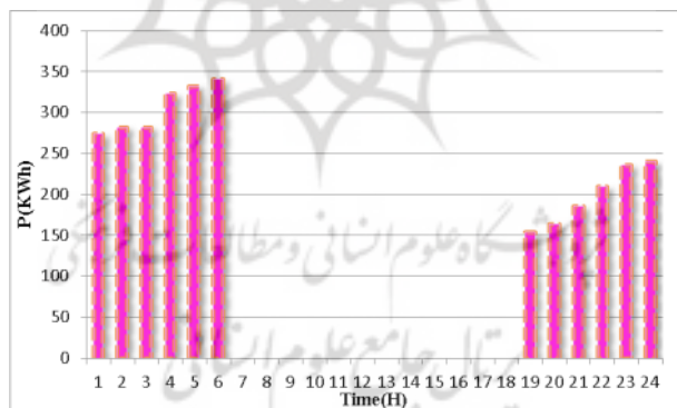
شکل ۱۵ سطح انرژی پارکینگ خودرو الکتریکی ۲
