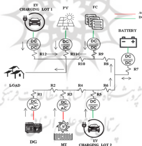
شکل ۱ ریز شبکه DC مورد نظر
