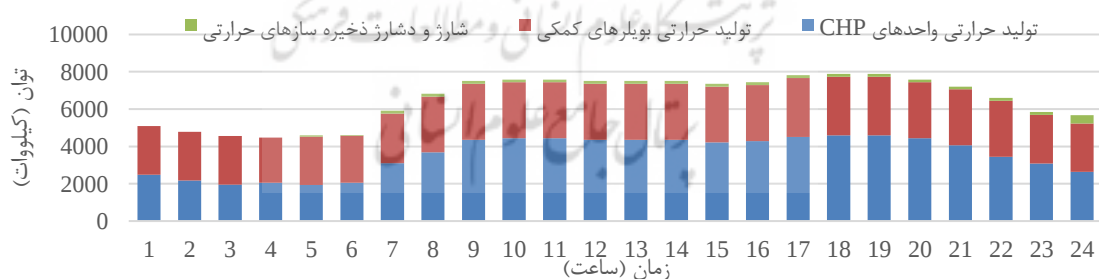
شکل ۱۲: تولید حرارتی منابع مختلف در شبکه ۱۸ شین برای ۲۴ ساعت در حالت سوم از دسته اول
