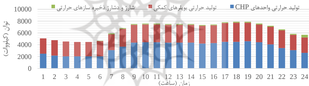
شکل ۲۱: تولید حرارتی منابع مختلف در شبکه ۱۸ شین برای ۲۴ ساعت در حالت ششم از دسته اول
