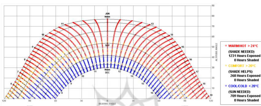
نمودار (۱۴) نمودار سازه‌ی سنجه از ابتدای تبر تا ابتدای دی (سنگری، ۱۳۹۹).
