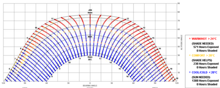
نمودار (۱۳) نمودار سازه‌سنجی از ابتدای دی تا ابتدای تیر (بگلی، ۱۳۹۹).
