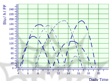
نمودار (۹) سطوح قائم (امتداد از جنوب 30°W) (بیگری، ۱۳۹۹).
