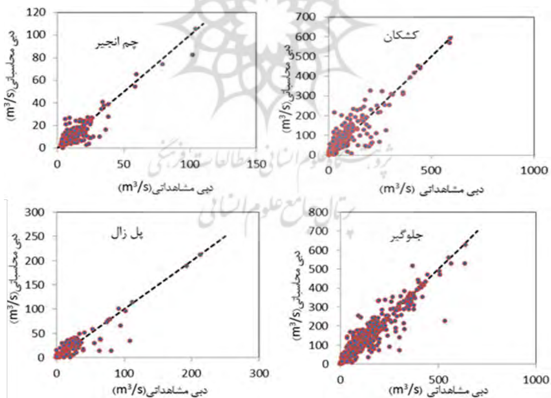
شکل (۷): نمودار پراکنش مقادیر مشاهده‌ای و محاسباتی مدل رگرسیون بردار پشتیبان-عنکبوت بیوه سیاه
