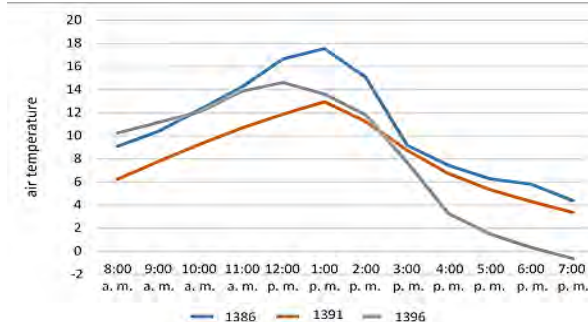
نمودار ۱. مقایسه دمای هوا در سه دوره
