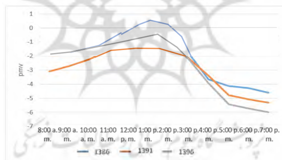
نمودار ۵. مقایسه میانگین آسایش حرارتی در سه دوره
