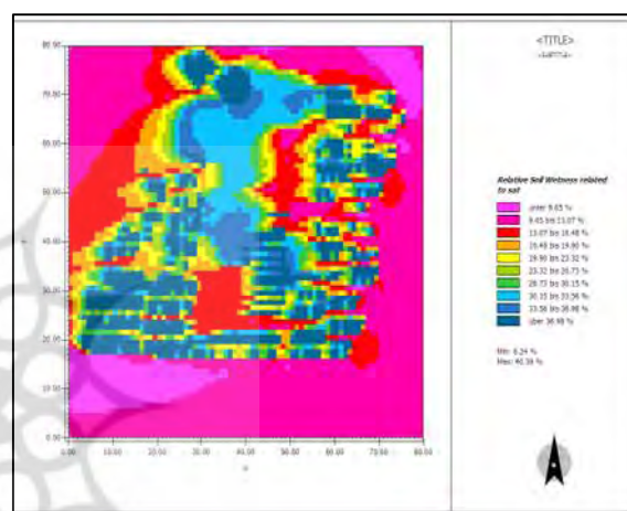
شکل ۱۳. میانگین رطوبت خاک روز ۱۳ بهمن ۱۳۹۶
