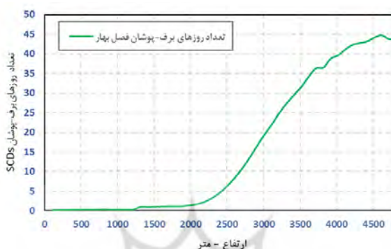
شکل ۱۱: پیوند تغییرات SCDs با سنج ارتفاع (فصل بهار)
