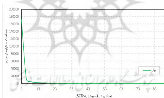
شکل ۷: پیوند SCAs با SCDs (فصل بهار)
