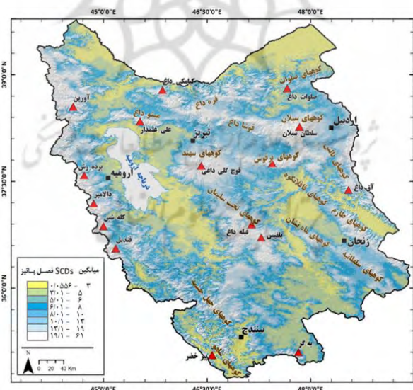
شکل ۵: میانگین فصلی SCDs در گستره شمال غربی ایران (پاییز)
