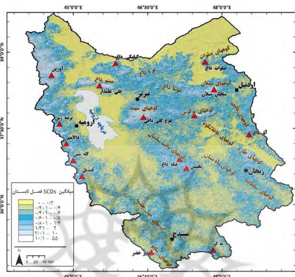
شکل ۴: میانگین فصلی SCDs در گستره شمال غربی (تابستان)
