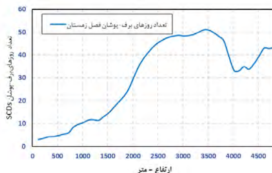
شکل ۱۰: پیوند تغییرات SCDs با سنج ارتفاع (فصل زمستان)
