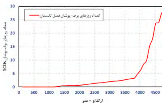
شکل ۱۲: پیوند تغییرات SCDs با سنج ارتفاع (فصل تابستان)
