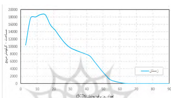
شکل ۶: پیوند SCAs با SCDs (فصل زمستان)
