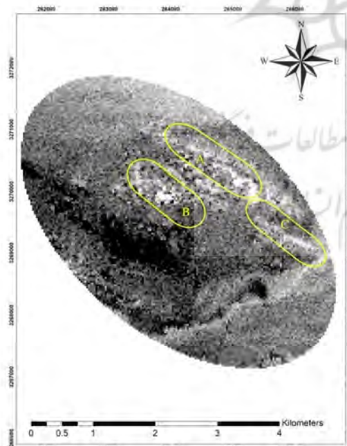
شکل ۱۲. تحلیل مؤلفه اصلی مربوط به PC3 آلتراسیون فیلک در منطقه مورد مطالعه
