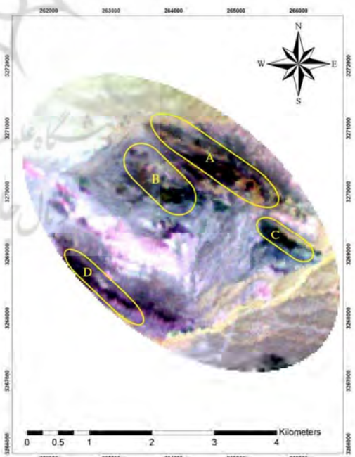
شکل ۸. ترکیب رنگی (۴۶۸) و آنومالی‌های احتمالی کانی‌زایی آهن‌دار در منطقه مورد مطالعه
