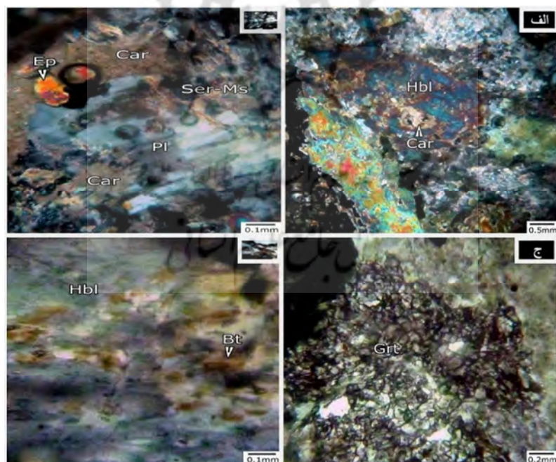
شکل ۳. مقطع میکروسکوپی نمونه (ب) محدوده مورد مطالعه: جانشینی کربنات در بلورهای پورفایروبلاست هورنبلاند (الف)؛ بقایای پلاژیوکلاز با جانشینی کربنات، سریسیت-موسکوویت و اپیدوت (ب)؛ نور (PPL) Plain Polarized Light نشان‌دهنده بلور پورفایروبلاست و انهدرال گارنت است (ج)؛ نمایی از بلورهای ریز بیوتیت در زمینه بلور پورفایروبلاست هورنبلاند که یافت پوئیکیلوبلاستیک را تشکیل داده است (د). علائم اختصاری در شکل: هورنبلاند = Hbl، کربنات = Car، اپیدوت = Ep، سریسیت و موسکوویت = Ser-Ms، بیوتیت = Bt و گارنت = Grt
