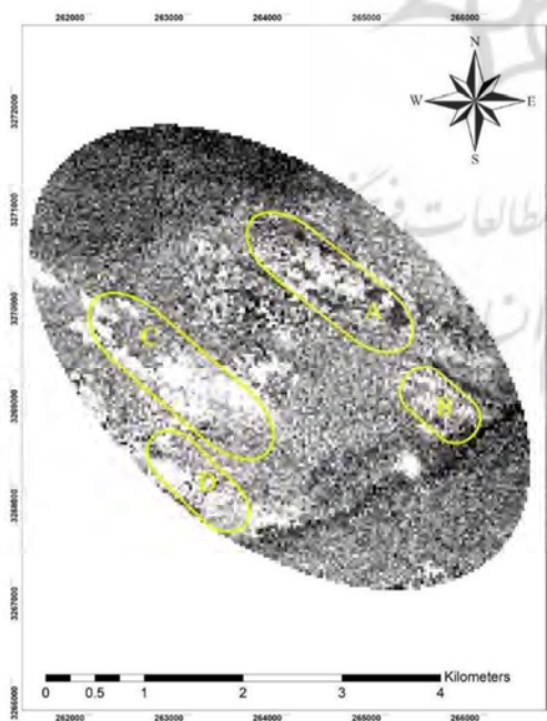
شکل ۱۰. نسبت‌گیری باندی ۶ / Band 6 (Band 5 + Band 7) و آنومالی‌های احتمالی کانی‌زایی آهن‌دار در منطقه مورد مطالعه
