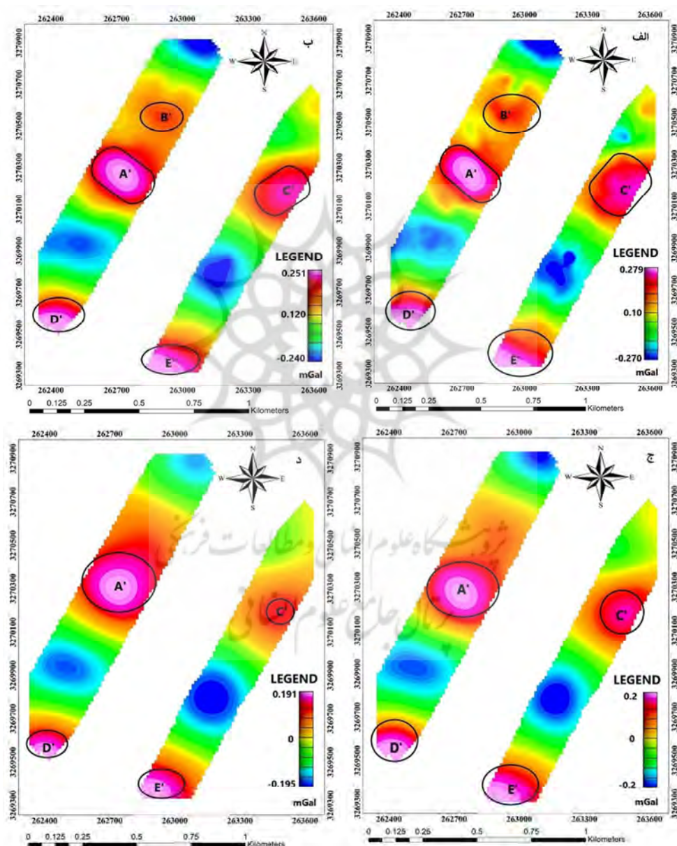
شکل ۱۸. نقشه‌های ادامه فراسو روی نقشه باقی‌مانده درجه دو گران‌سنجی زمینی؛ نقشه ادامه فراسو با ارتفاع ۱۰ متر از سطح زمین (الف)؛ نقشه ادامه فراسو با ارتفاع ۵۰ متر از سطح زمین (ب)؛ نقشه ادامه فراسو با ارتفاع ۸۰ متر از سطح زمین (ج)؛ نقشه ادامه فراسو با ارتفاع ۱۰۰ متر از سطح زمین در محدوده مورد مطالعه (د)
