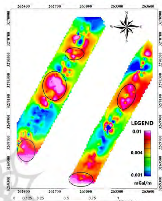
شکل ۱۹. نقشه مشتق قائم مرتبه اول روی نقشه باقی‌مانده درجه دو گرانی‌سنجی زمینی در محدوده مورد مطالعه
