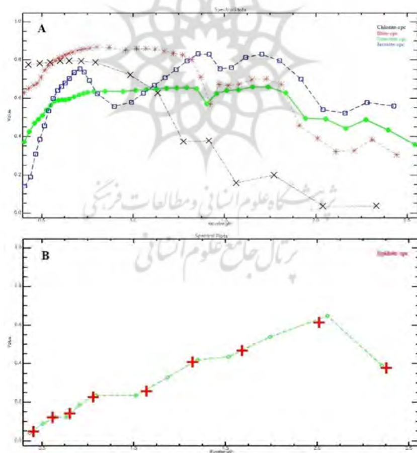
شکل ۱۳. نمودار نقشه‌برداری زاویه طیفی و پراکندگی کانی‌های کلریتی، ایلیتی، اسمکتیتی و ژاروسیت (A)؛ نمودار نقشه‌برداری زاویه طیفی کانی‌سازی اپیدوتی در منطقه مورد مطالعه (B)
