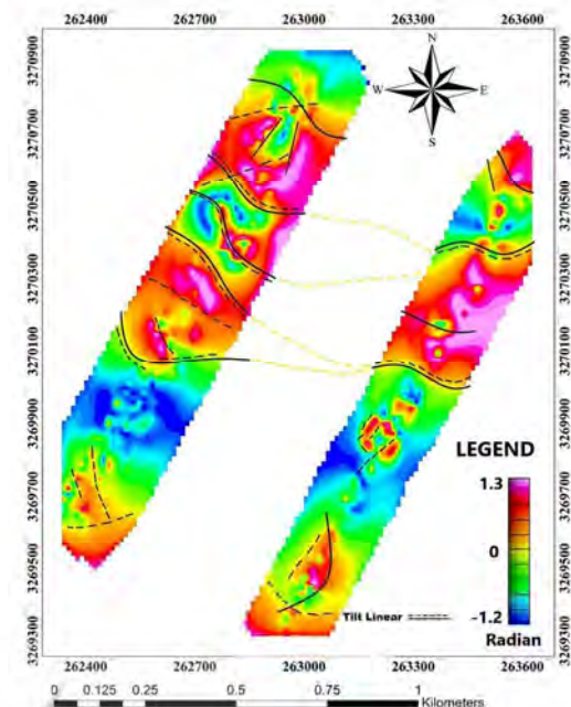
شکل ۲۱. نقشه زاویه تمایل به همراه خطواره‌های استخراج شده روی نقشه باقی‌مانده درجه دو گرانی‌سنجی زمینی در محدوده مورد مطالعه
