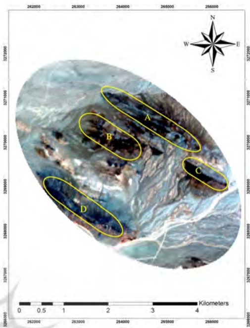
شکل ۷. ترکیب رنگی (۱۲۳) و آنومالی‌های احتمالی کانی‌زایی آهن‌دار در منطقه مورد مطالعه
