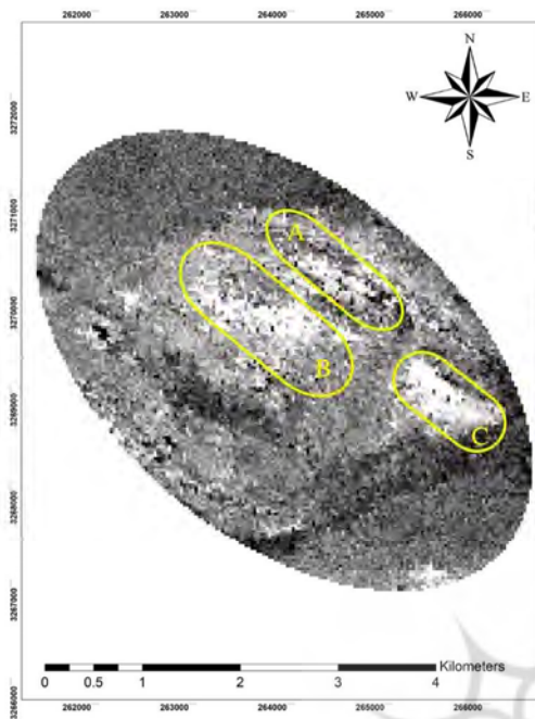
شکل ۹. نسبت‌گیری باندی ۵ / Band 4 و آنومالی‌های احتمالی کانی‌زایی آهن‌دار در منطقه مورد مطالعه
