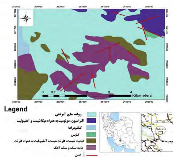
شکل ۱. نقشه زمین‌شناسی منطقه مورد مطالعه
