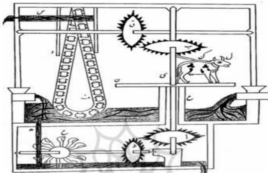
تصویر ۹. دستگاه سوم جزری صفحه ۴۶۲ کتاب الجامع بین العلم والعمل النافع فی صناعة الحیل تصحیح احمد یوسف حسن
