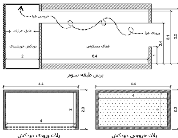
تصویر ۶. جزئیات دودکش خورشیدی. مأخذ: نگارندگان.
