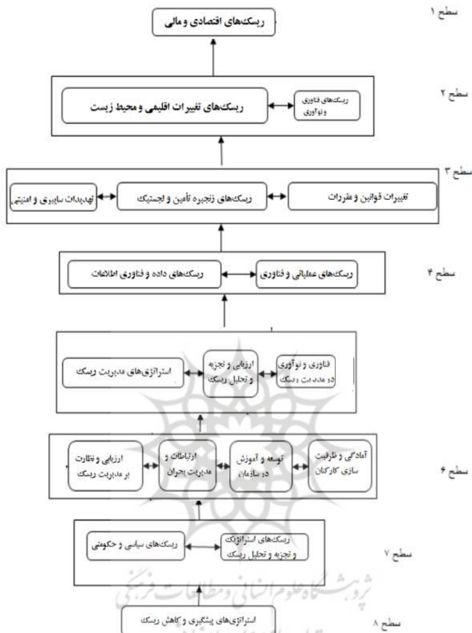
شکل ۳: مدل استراتژی‌های مواجهه با ریسک‌های اولویت دار در عملیات پالایشگاه نفت
