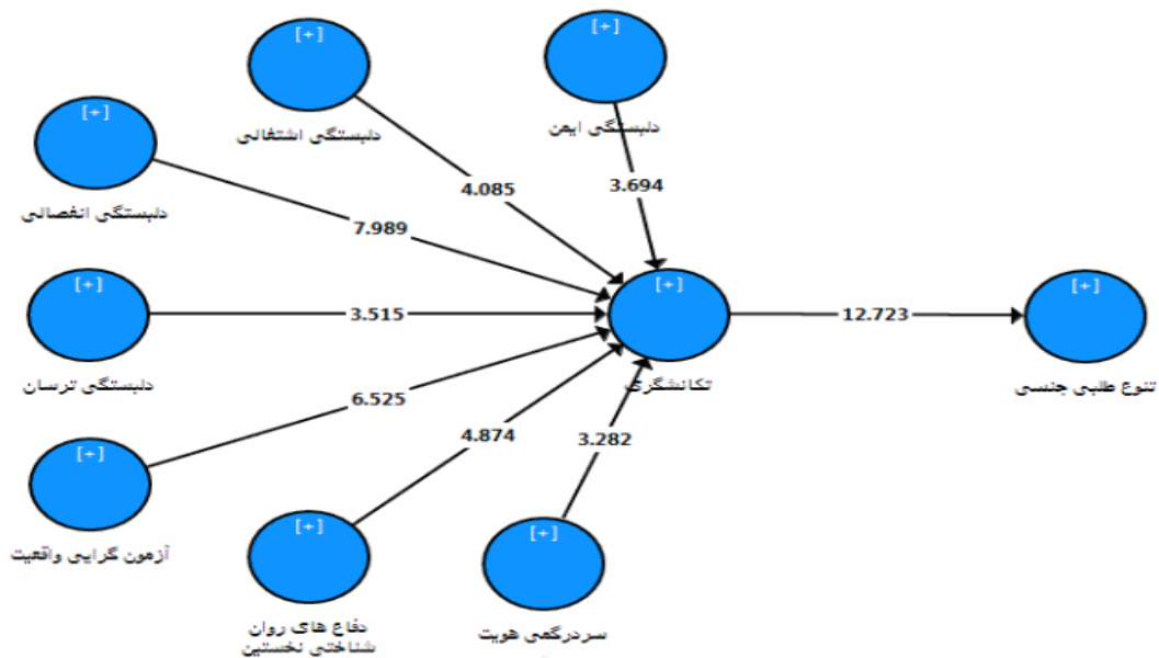
شکل ۲. نتایج آزمون تی - استیوودنت برای بررسی معناداری ضرایب مسیر
