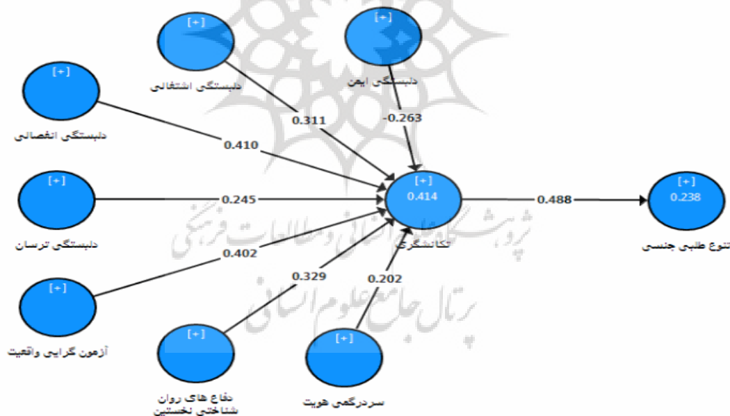
شکل ۱. ضرایب مسیر استاندارد مدل مفهومی پژوهش
