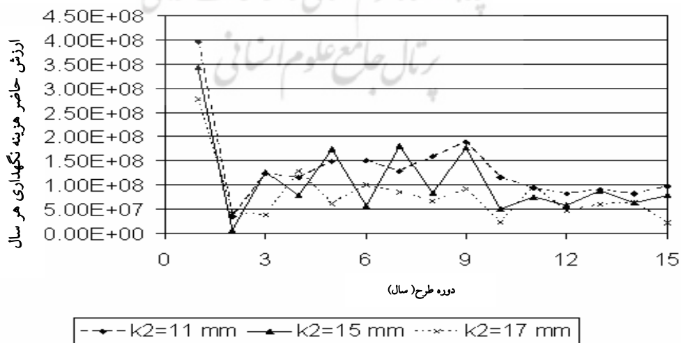
شکل 9. نمودار ارزش حاضر هزینه‌های سالانه برای چند سطح هشدار خرابی شیارشستگی
