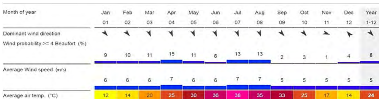
شکل ۱. جهت و میانگین سرعت باد و دما در ماه‌های مختلف سال در شهر یزد
