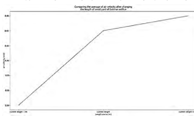
شکل ۱۴. تاثیر طول بر سرعت هوا در حیاط کوچک خانه گلشن
