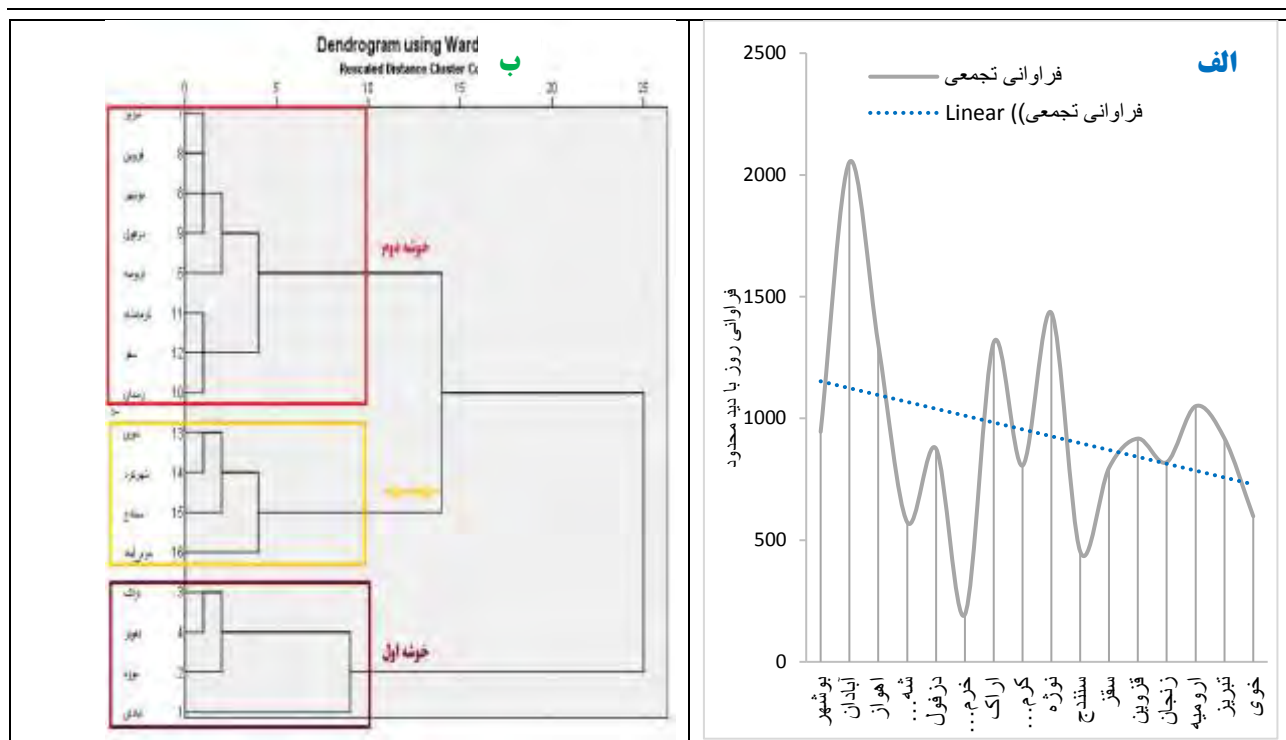
شکل (۲): نمودار فراوانی روزهای با دید محدود دوره (الف) و خوشه‌بندی ایستگاه‌ها برحسب آن (ب)
