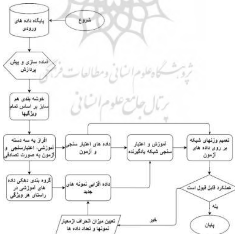
شکل (۲): فلوچارت روش ارائه شده جهت داده افزایشی مقید بر مبنای عملکرد
