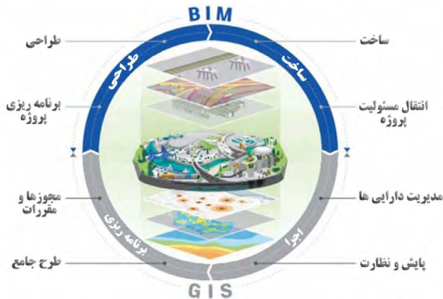
شکل ۳. چرخه یکپارچه سازی GIS و BIM
