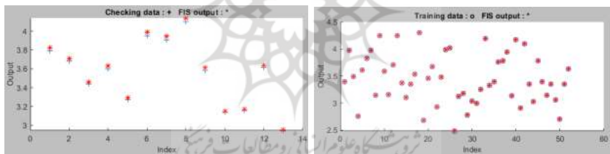
شکل ۵. مقایسه بین خروجی ANFIS و داده‌ها - سمت راست) داده‌های آموزش؛ سمت چپ) داده‌های اعتبارسنجی
